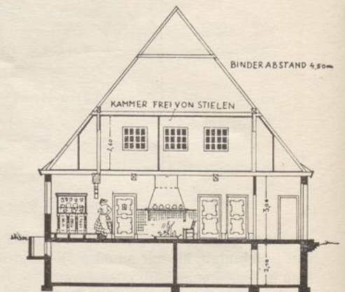
WOHNTEIL-QUERSCHNITT (VERSPRUNGEN)
