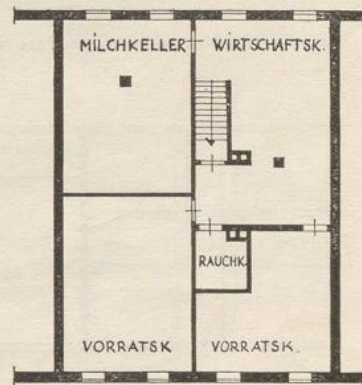
KELLERGESCHOSS
