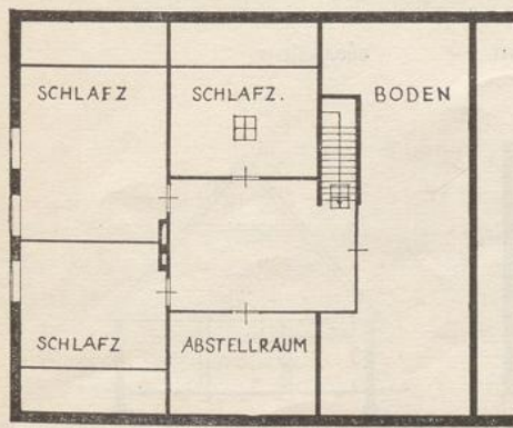
AUSGEB. DACHGESCHOSS
