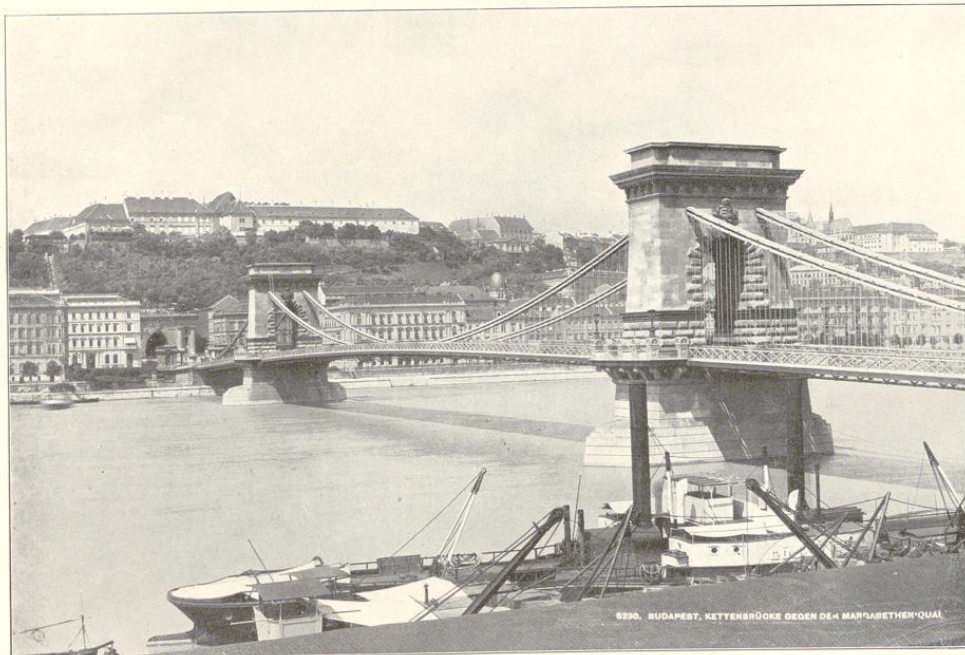
Abb. 87. Kettenbrücke in Budapest. 1839–45. Nach Photographie Alois Beer, k. u. k. Hof- u. Marine-Photograph, Klagenfurt 1908.
