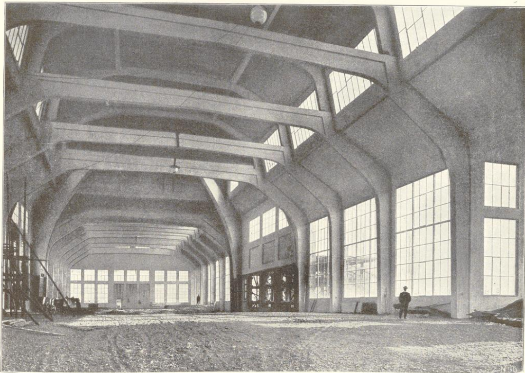
Abb. 162. Halle (mit Eisenbetonbindern) im Ausstellungspark in München. Nach: „E. von Mecnseff, Die künstlerische Gestaltung der Eisenbetonbauten.“ Verlag von Wilhelm Ernst & Sohn, Berlin.
