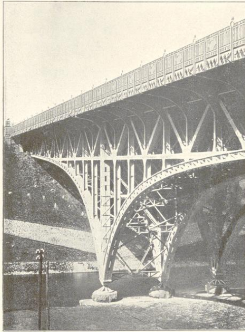
Abb. 79. Schrägaussicht der Stössenseebrücke bei Spandau. 1908.
