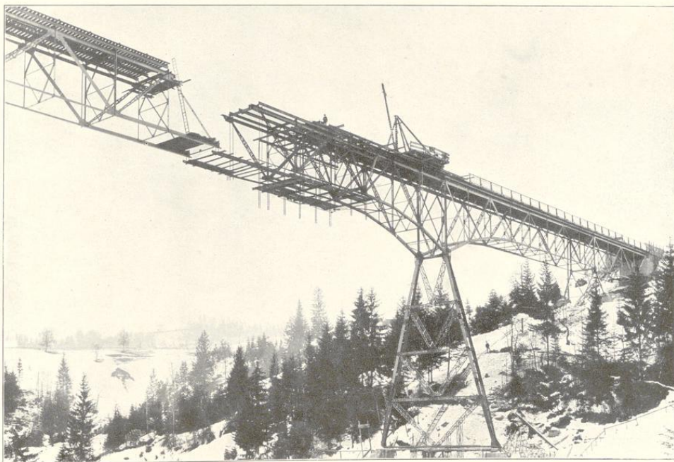
Abb. 40. Brücke über den Argentobel. 1905—07. Nach Abb. der Maschinenfabrik Augsburg-Nürnberg, A.-G., Werk Gustavsburg.
