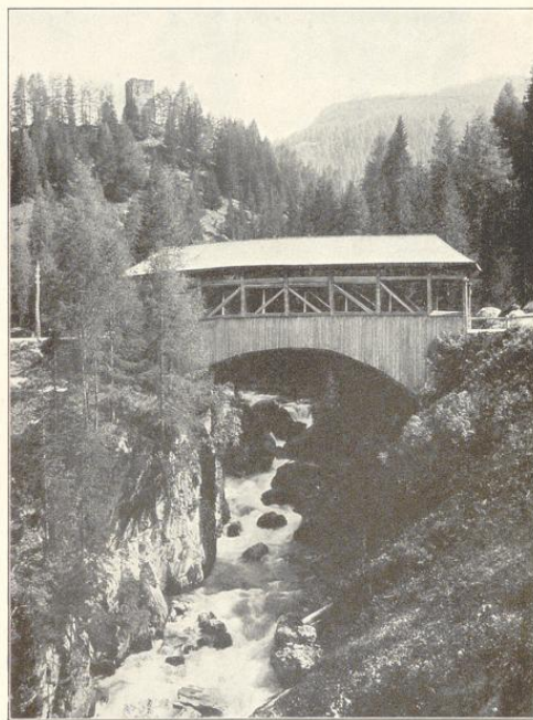
Abb. 110. Überdeckte Holzbrücke. Brücke an der Julierstraße bei Mühlent. Nach: „Denkmalpflege“ 1911, S. 11. Verlag von Wilhelm Ernst & Sohn, Berlin.
