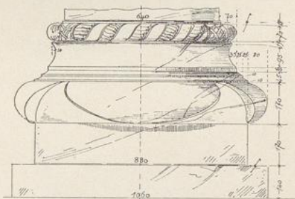
Fig. 147. Kapitell. Hildesheim. St. Michael. Mittelschiff. Aus der Zeit Adolgs. (XII. Jahrh.)
