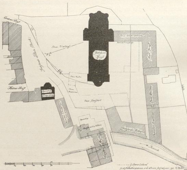
Fig. 171. Hildesheim. St. Godehard. Lageplan.
