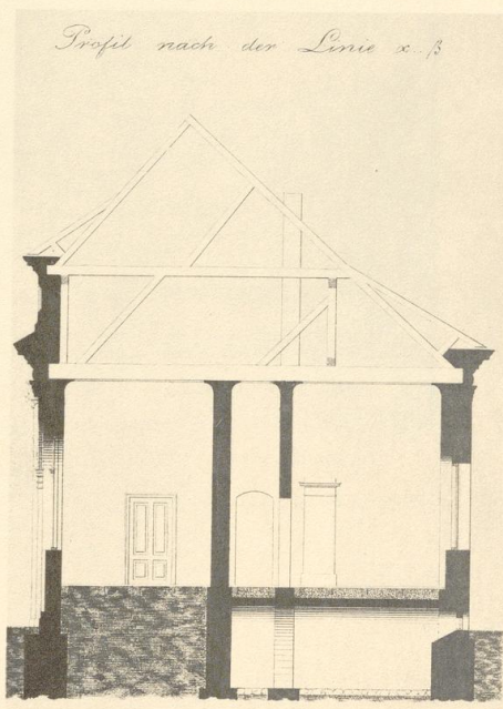
89.—91. Das 1685 erbaute halbovale Pomeranzenhaus, Zeichnungen aus dem Jahre 1832 mit damals geänderter Raumbenutzung
