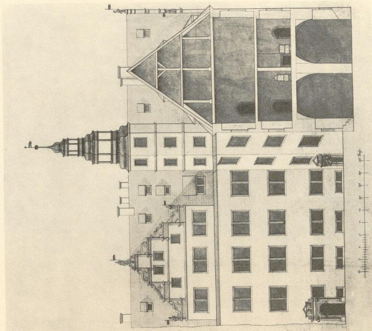
71. Schloß Dessau, Querschnitt durch den südlichen Flügel
