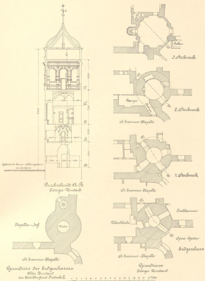
9. Der „Grüne Hut“ in Grundrissen und Schnitt
