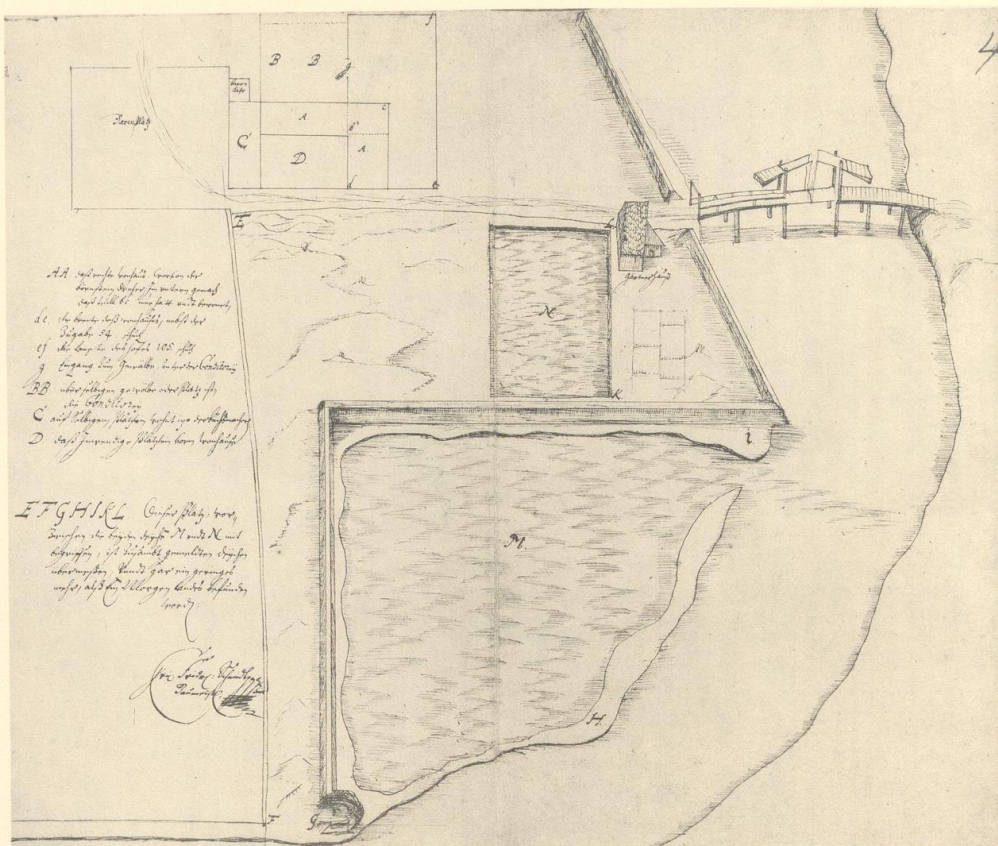
74. Lageplan eines Teiles des Cölnischen Werders, von dem Baumeister Christoph Friedrich Schmidt, 1643
