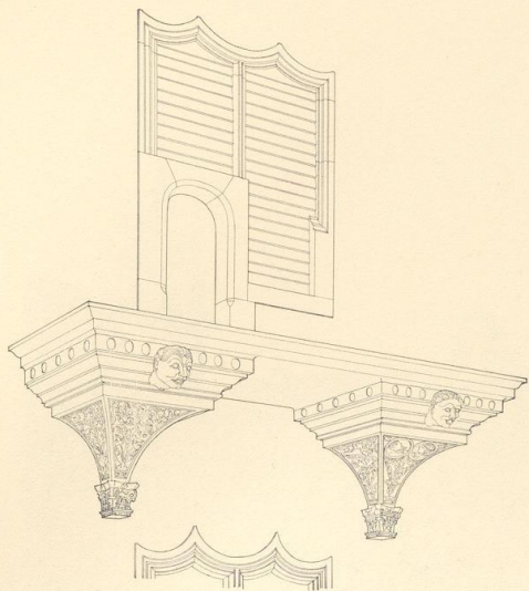
34. Balkonrest am Kapellenturm, Zeichnung nach Aufmessung
