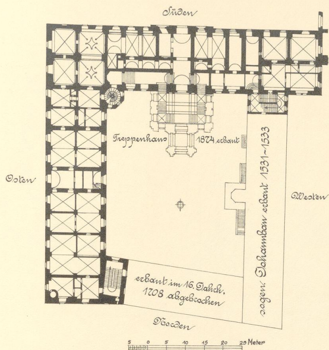
69. Erdgeschoß des vom Grafen zu Linar entworfenen und erbauten Ost- und Südflügels des Schlosses zu Dessau, 1574—1578
