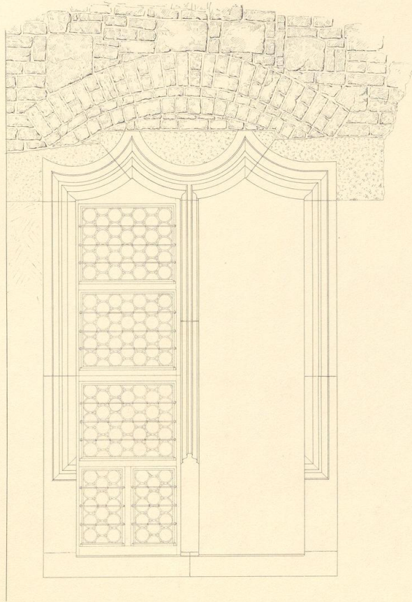
34. Balkonrest am Kapellenturm, Zeichnung nach Aufmessung
