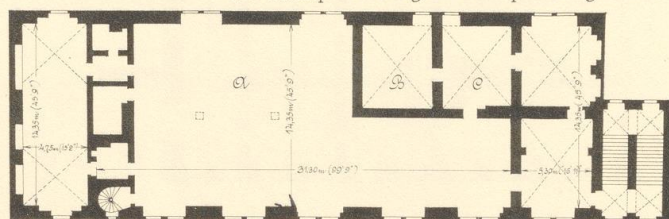
Grundriss des Ober-Geschosses Nach alten Grundrissen aus dem Jahre 1579
