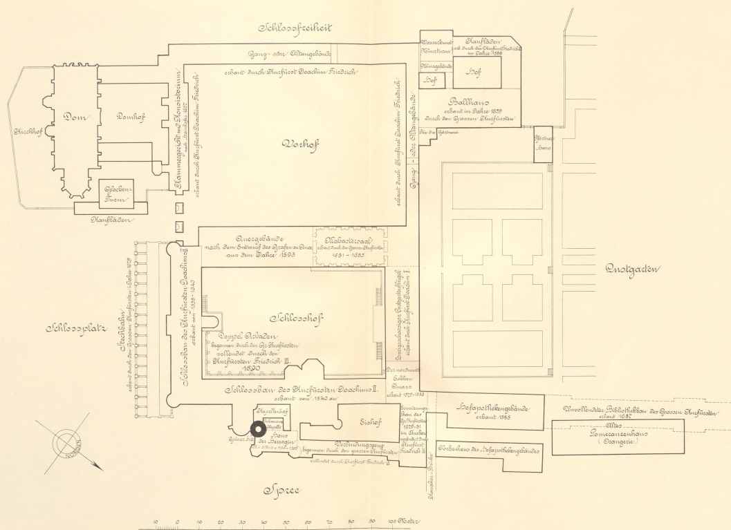
154. Umrissplan des Schloßbaus zur Zeit des Großen Kurfürsten und des Kurfürsten Friedrich III. bis zum Beginn des Umbaus durch Schlüter, 1698
