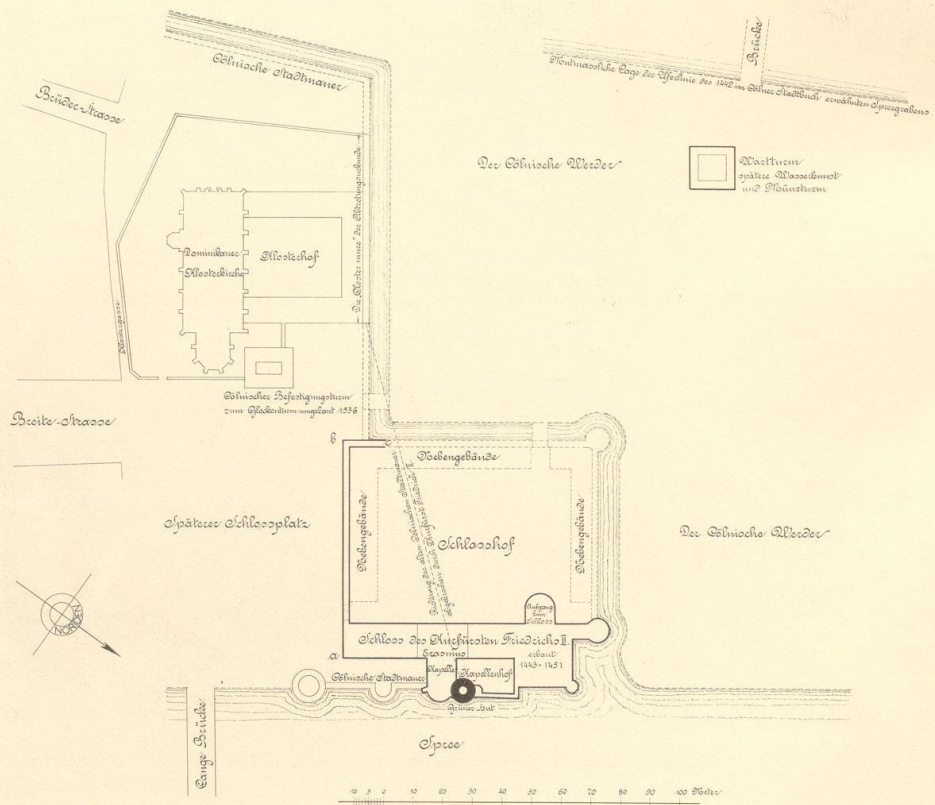
13. Umrissplan des Schloßbaus Kurfürst Friedrichs II. auf Grund der Mauerwerksuntersuchung
