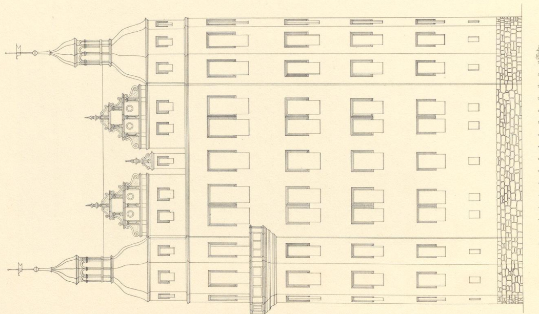
63. Das Haus der Herzogin, Wiederherstellung der ursprünglichen Ansicht nach der Spree
