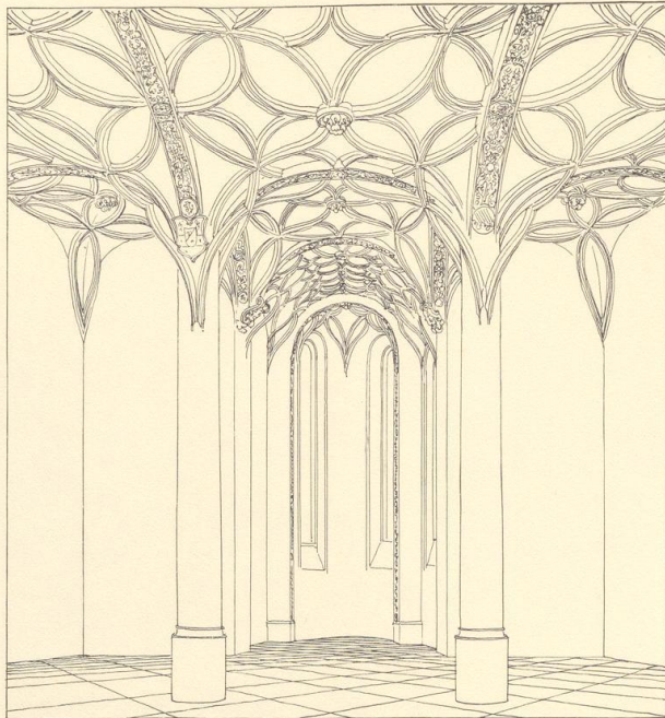
42. Der Innenraum der St. Erasmus-Kapelle in ganzer Höhe nach Aufmessung. Lichte Höhe 13,17 m
