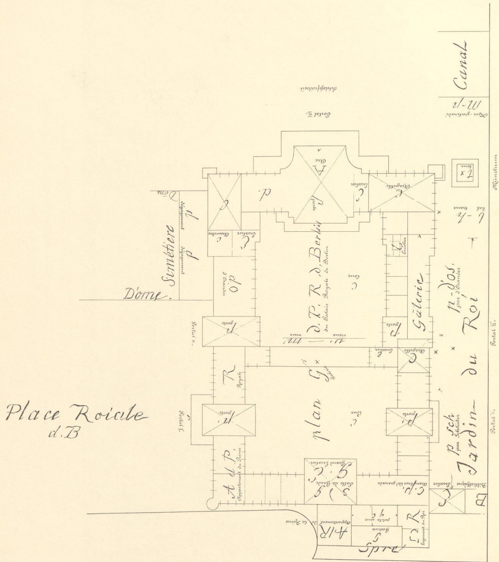
116. Vergrößerter Übersichtsplan des Schlosses nach Broches (1733), mit Erklärung der Buchstabenbezeichnungen
