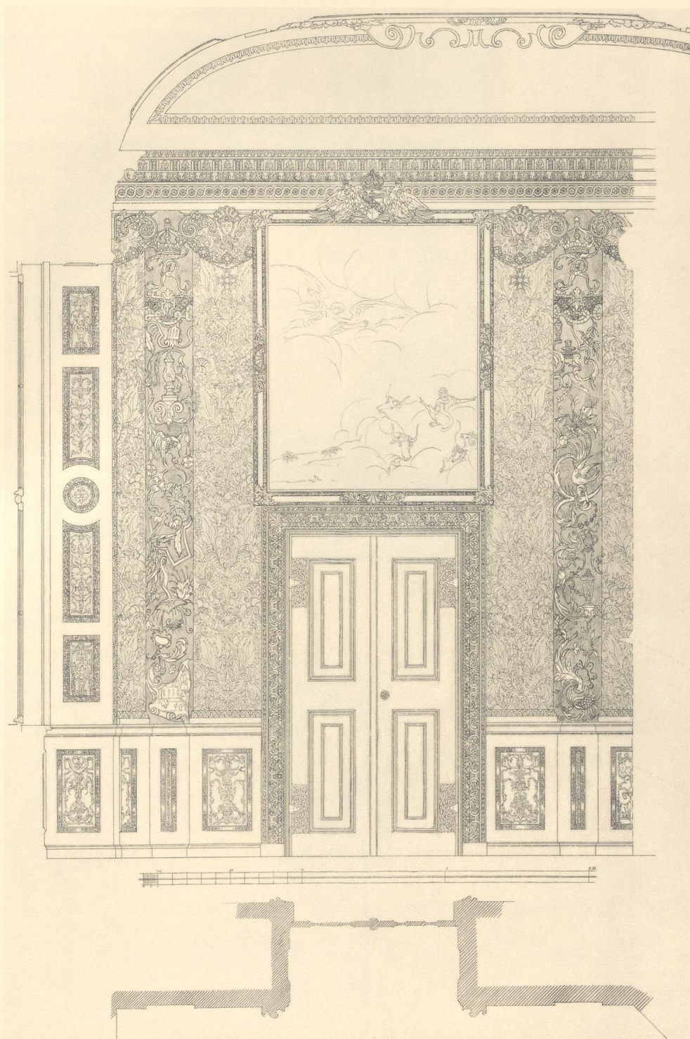
107. Ansicht der nordöstlichen Schmalwand in Raum 5 der Wohnung des Großen Kurfürsten nach dem Ausbau durch Schlüter nach 1701
