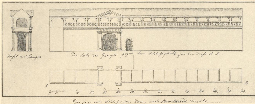
20. Entwurf von J. G. Memhardt für einen Neubau des Ganges vom Schloßplatzflügel zum Dom über dem Haupteingang zum Schloß hinweg
