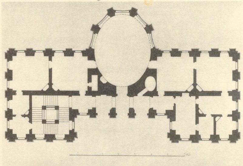
150. Grundriß des Schlosses Lietzenburg nach dem Umbau durch Schlüter
