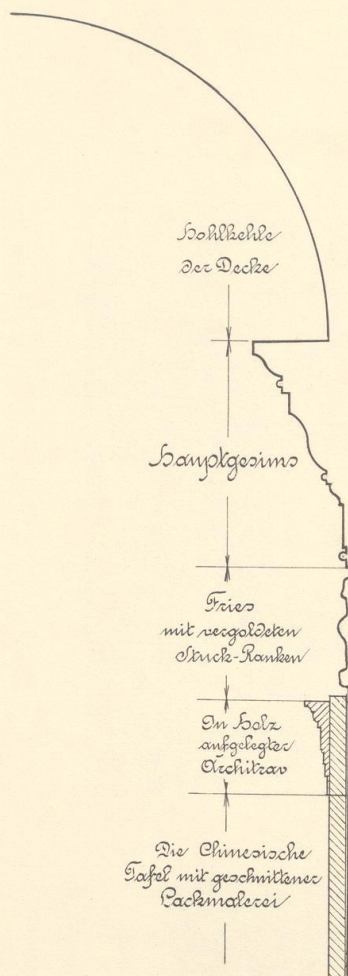
126. Schnitt durch das Gesims im jetzigen „Chinesischen Cabinet“ C
