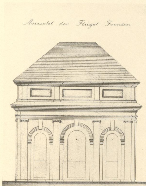
89.—91. Das 1685 erbaute halbovale Pomeranzenhaus, Zeichnungen aus dem Jahre 1832 mit damals geänderter Raumbenutzung
