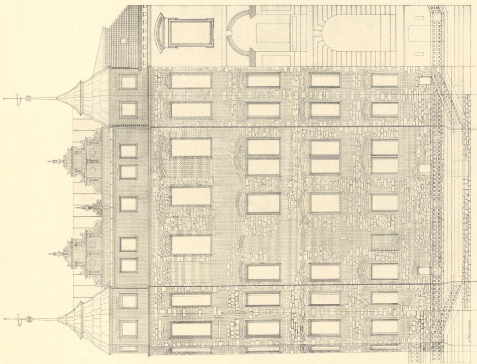
61. Aufnahme-Zeichnung der Ansicht des Hauses der Herzogin nach der Spree, vor dem Neuabputz
