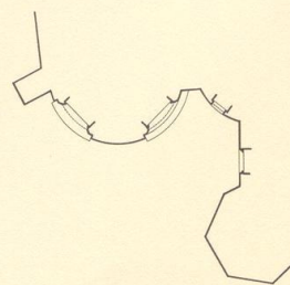
32. Die Spreefront des Kapellenturms mit Ergänzung der abgebrochenen Endigung
