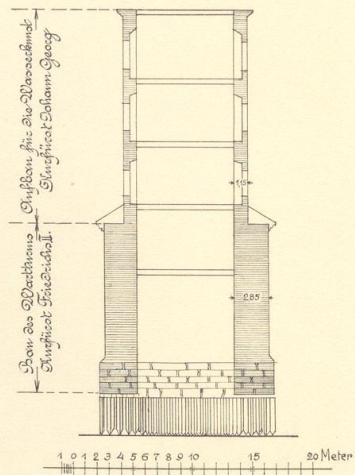
76. Schnitt durch den Turm der „Neuen Wasserkunst“ auf dem alten „Wartturm“ Kurfürst Friedrichs II.
