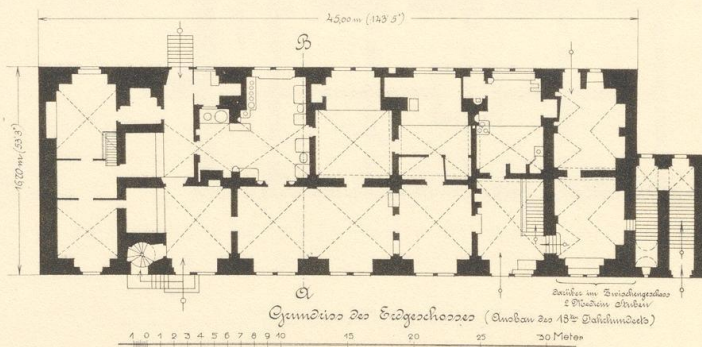
57. Die zwei Grundrisse des Hofapothekeengebäudes
