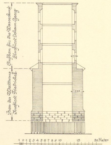
76. Schnitt durch den Turm der „Neuen Wasserkunst“ auf dem alten „Wartturm“ Kurfürst Friedrichs II.
