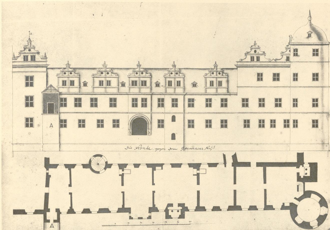
19. Stadtansicht des Schlosses Küstrin mit dem Ausgang des „hultzen gangks“ zur Stadtkirche bei A im Schnitt und Grundriß
