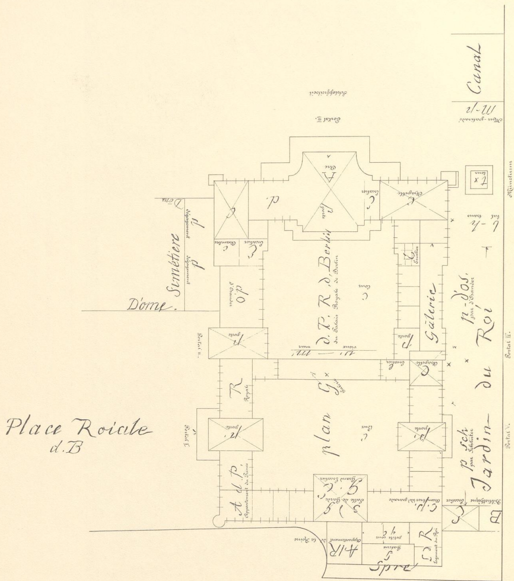
116. Vergrößerter Übersichtsplan des Schlosses nach Broebes (1733), mit Erklärung der Buchstabenbezeichnungen
