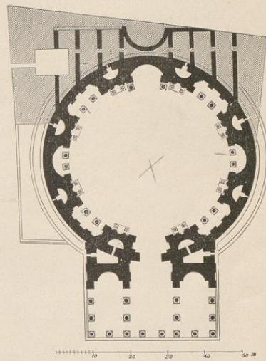
5. Grundriss des Pantheons. Die hinter der Rotunde angegebenen Bauteile gehören einer älteren Anlage an.
