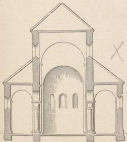
9. Querschnitt einer romanischen Basilika.
