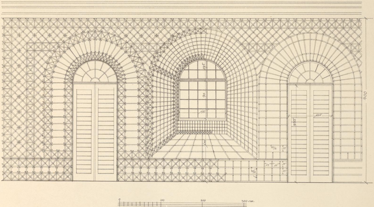
Spalier am Stallgebäude Wien, Praterstraße.
