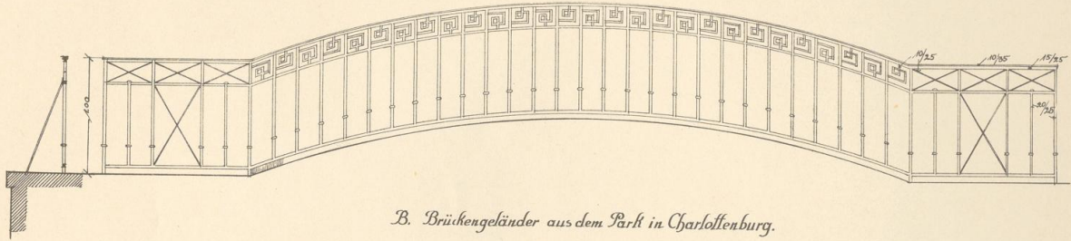
A. Brückengeländer aus dem Park in Charlottenburg.
