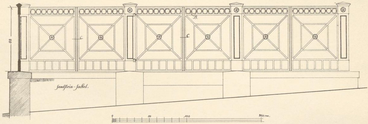
Erbgrabmal auf dem alten Friedhof in Eisenach. Kugeln, Perlstab u. Bund B. vergoldet.
