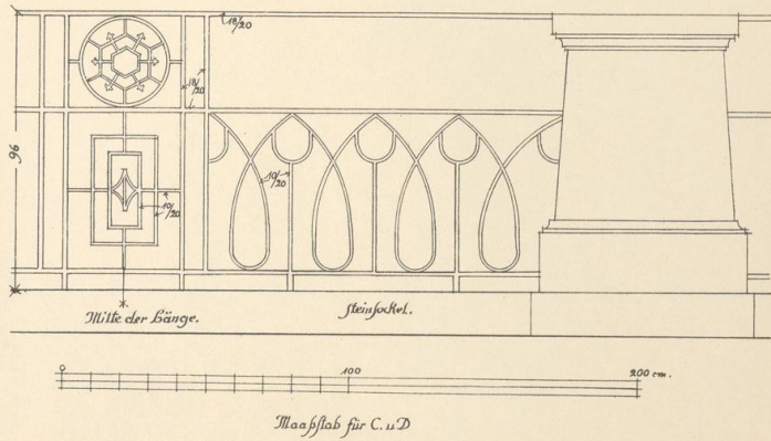
D. Brückengeländer aus Potsdam
