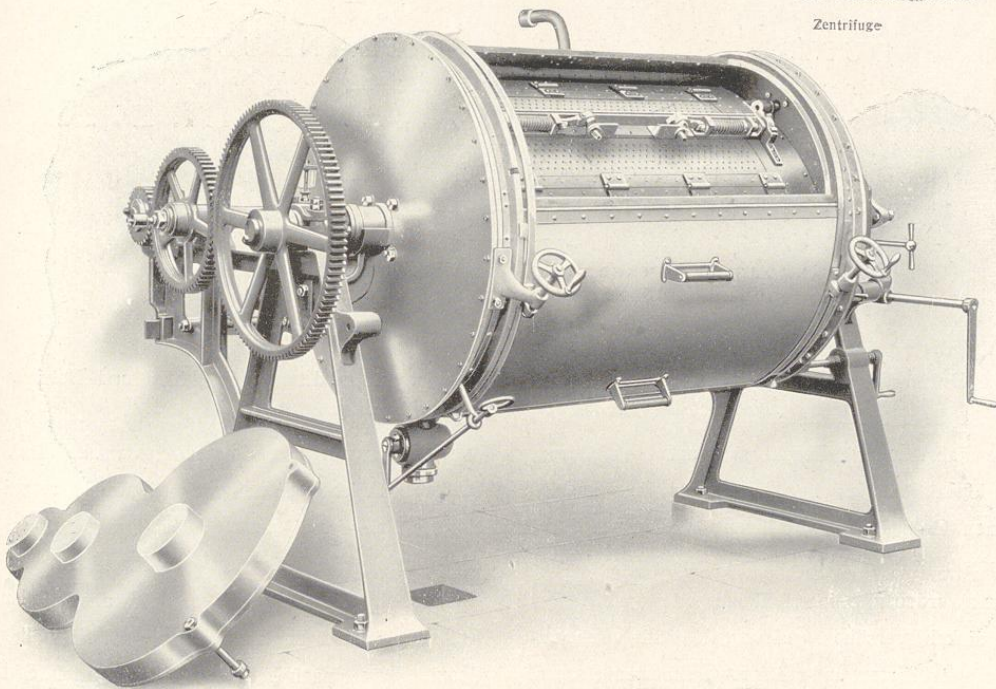
Kippbare Dampfwaschmaschine mit hintenliegendem Antrieb
