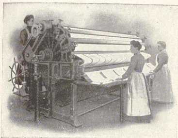
Zylinder-Dampfmangel
