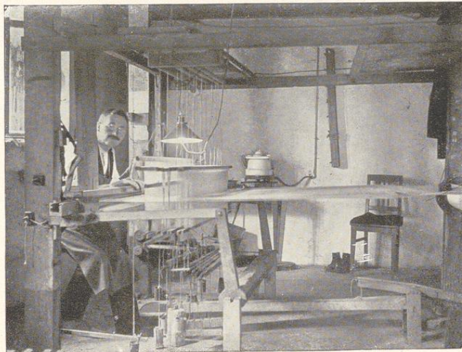
Seidenbeutelweber bei der Arbeit. — Echte Schweizer Müllergaze muß noch sorgfältig mit der Hand in Kellern hergestellt werden, letzteres, weil zum Weben eine möglichst gleichbleibende Feuchtigkeit der Luft nötig ist
