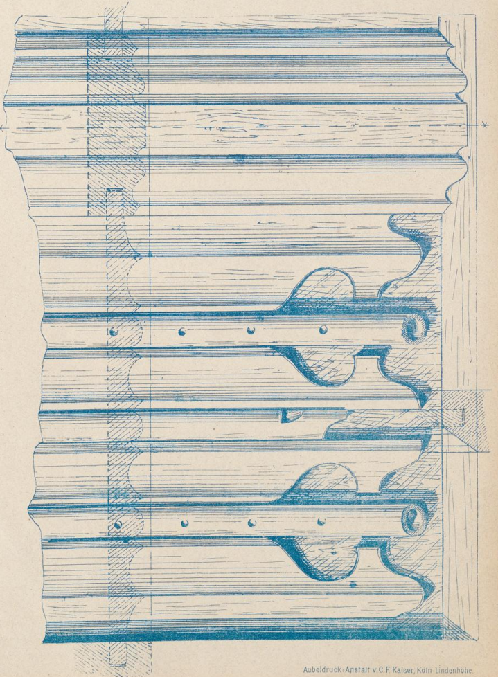
DETAILS in nat. Gr. zum STOLLENSCHRANK Taf. No. 2 A
