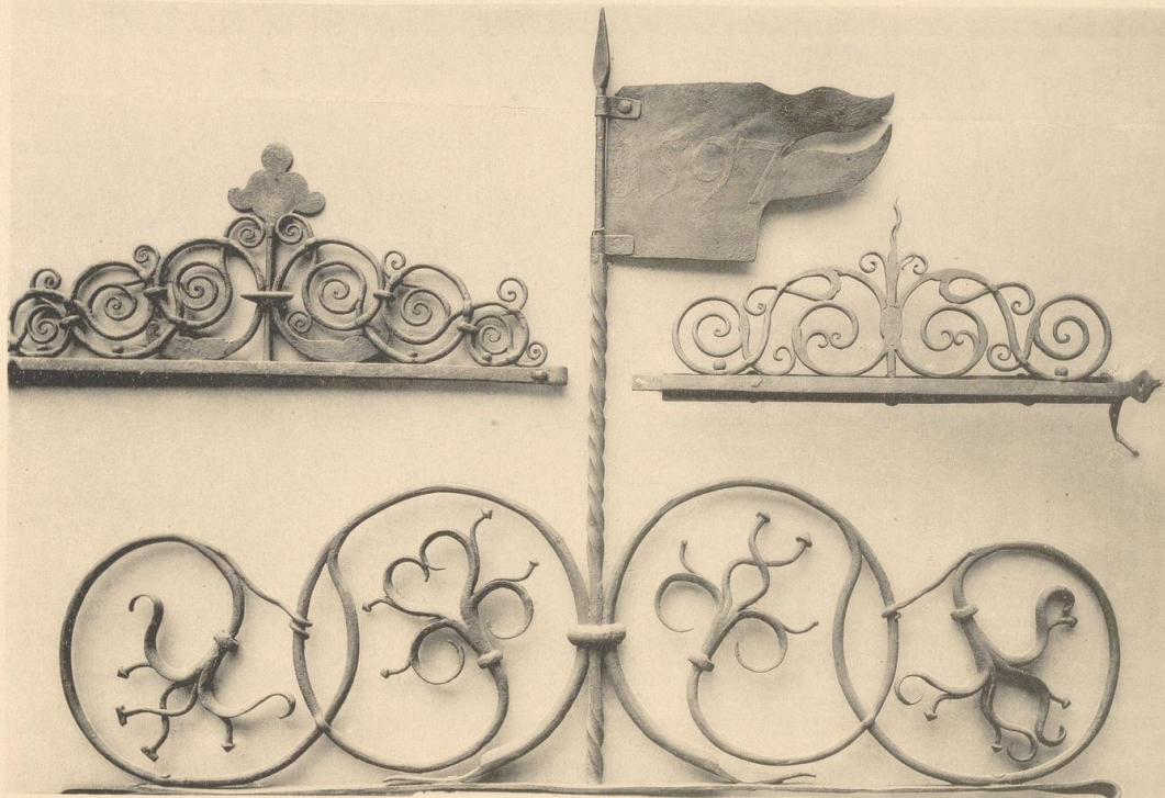
Bekrönungen aus gebogenem und geschmiedetem Rundeisen. 16. u. 17. Jahrhundert. Germanisches Museum in Nürnberg.
