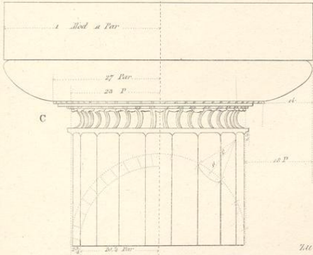
Profil der Säule C.
