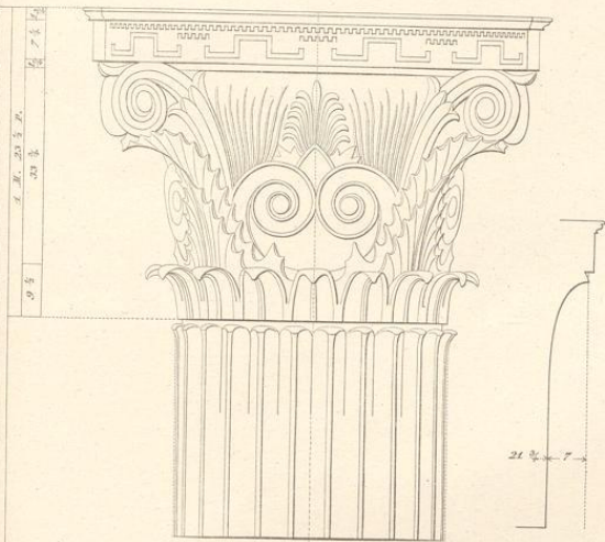
Säule, aus dem Inneren des Apollo Tempels zu Bassæ.
