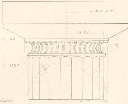
Profil der Säule D.
