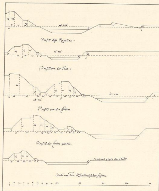
Abb. 20. Die Profile der Befestigungswerke der Zitadelle, um 1680? (Verzeichnis Nr. 63, Pause)
