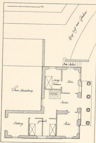
Abb. 52. Grundriß des Torschreiberhauses am Max-Tor von W. F. Lipper, um 1780 (Verzeichnis Nr. 135, Pause)
