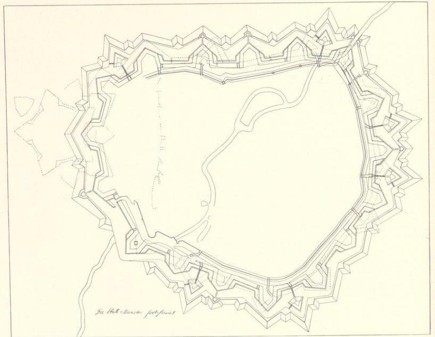
Abb. 26. Entwurf einer Neubefestigung, um 1683 (Verzeichnis Nr. 71, Pause)
