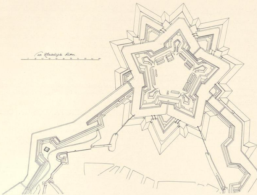
Abb. 31. Vogelschau-Entwurf einer Neubefestigung, 1688 (Verzeichnis Nr. 77, Pause)
