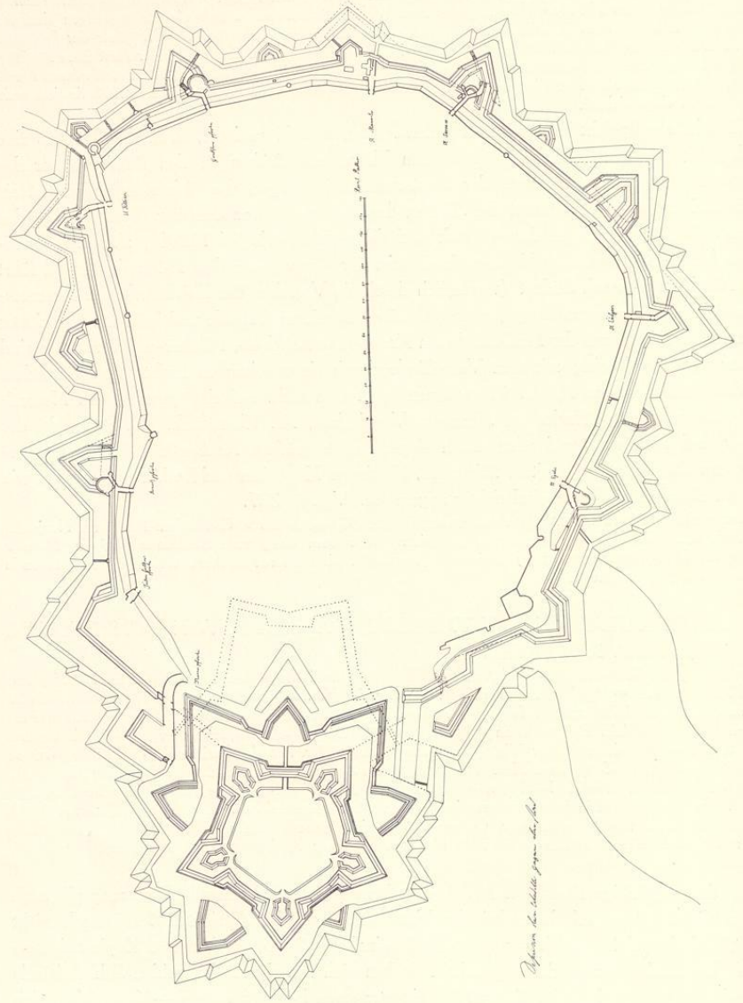
Abb. 34. Entwurf einer Verstärkung der Stadtbefestigungen, 1689 (Verzeichnis Nr. 82, Pause)
