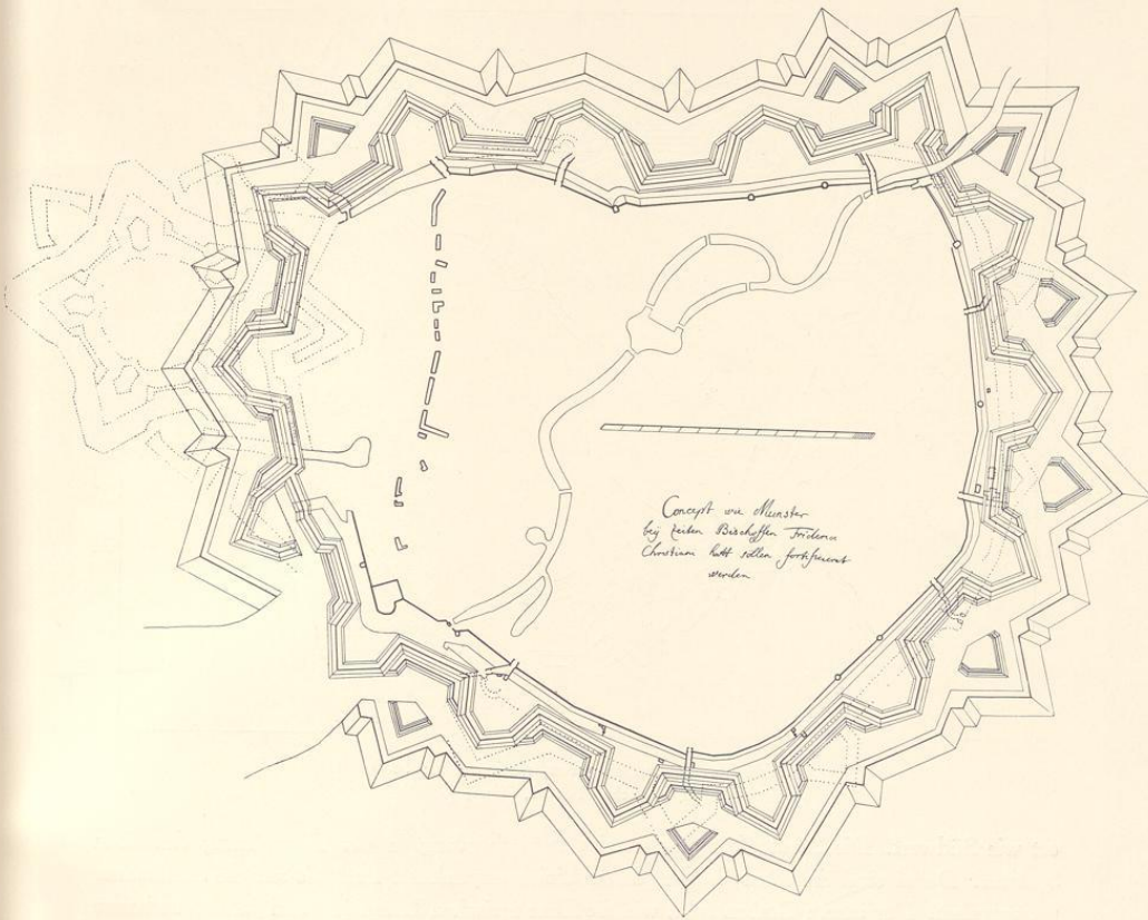
Abb. 25. Entwurf einer Neubefestigung, um 1683 (Verzeichnis Nr. 70, Pause)
