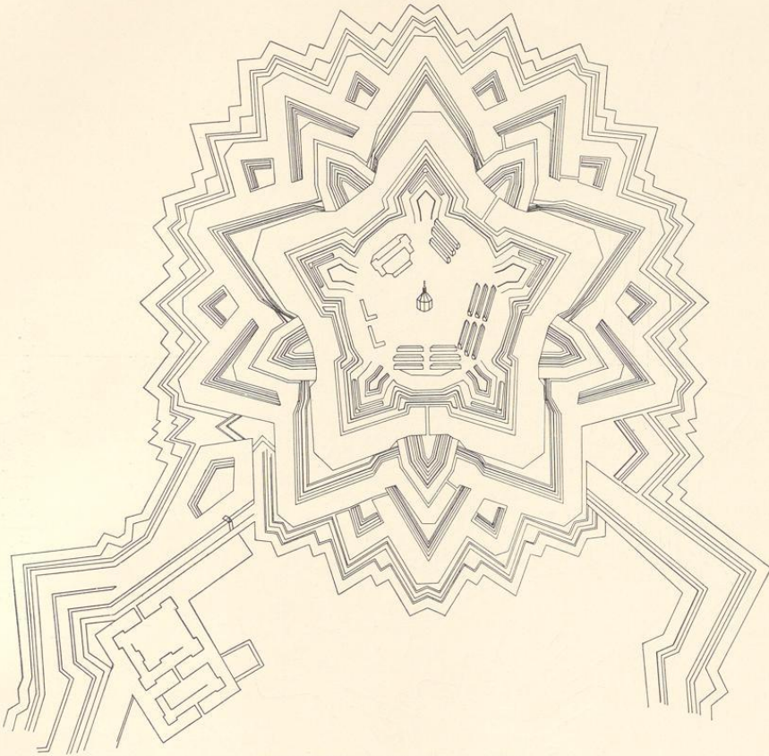
Abb. 18. Plan der Zitadelle, um 1680 (Verzeichnis Nr. 60, Pause)
