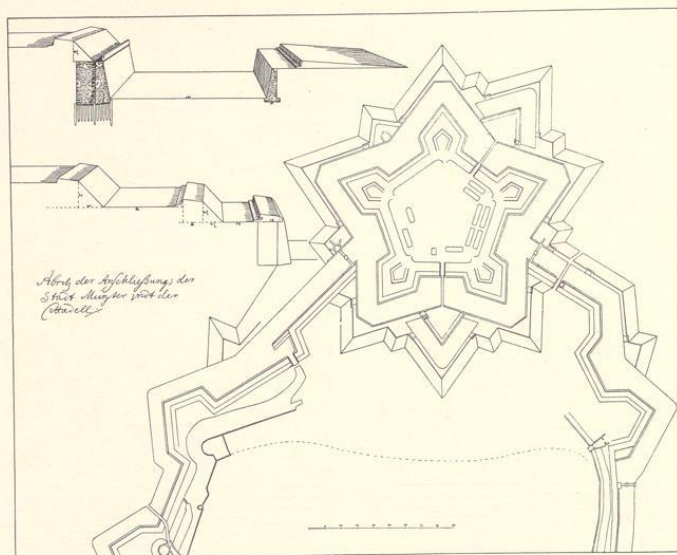
Abb. 30. Entwurf der Befestigung der Zitadelle mit Eskarpen, 1685 (Verzeichnis Nr. 75, Pause)
