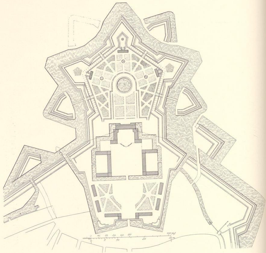
Abb. 42. Entwurf einer Residenz mit Schloßgarten, Schloßplatz und Hornwerk, um 1733 (Verzeichnis Nr. 91, Pause)
