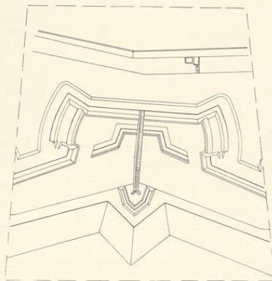
Abb. 27. Entwurf eines Teiles der Neubefestigung (Verzeichnis Nr. 72, Pause)
