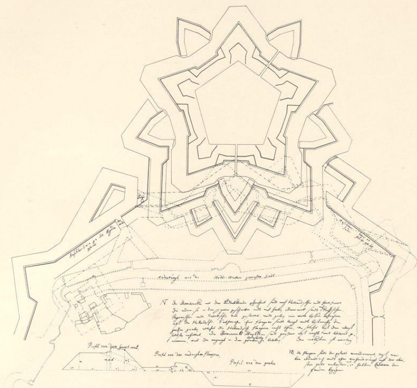
Abb. 21. Entwurf einer Neubefestigung, um 1680 (Verzeichnis Nr. 64, Pause)
