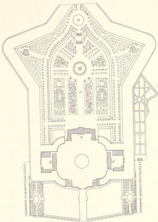
Abb. 48. Entwurf der Schloßanlage, um 1771 (Deckblatt zu Nr. 84; Verzeichnis Nr. 118, Pause)
