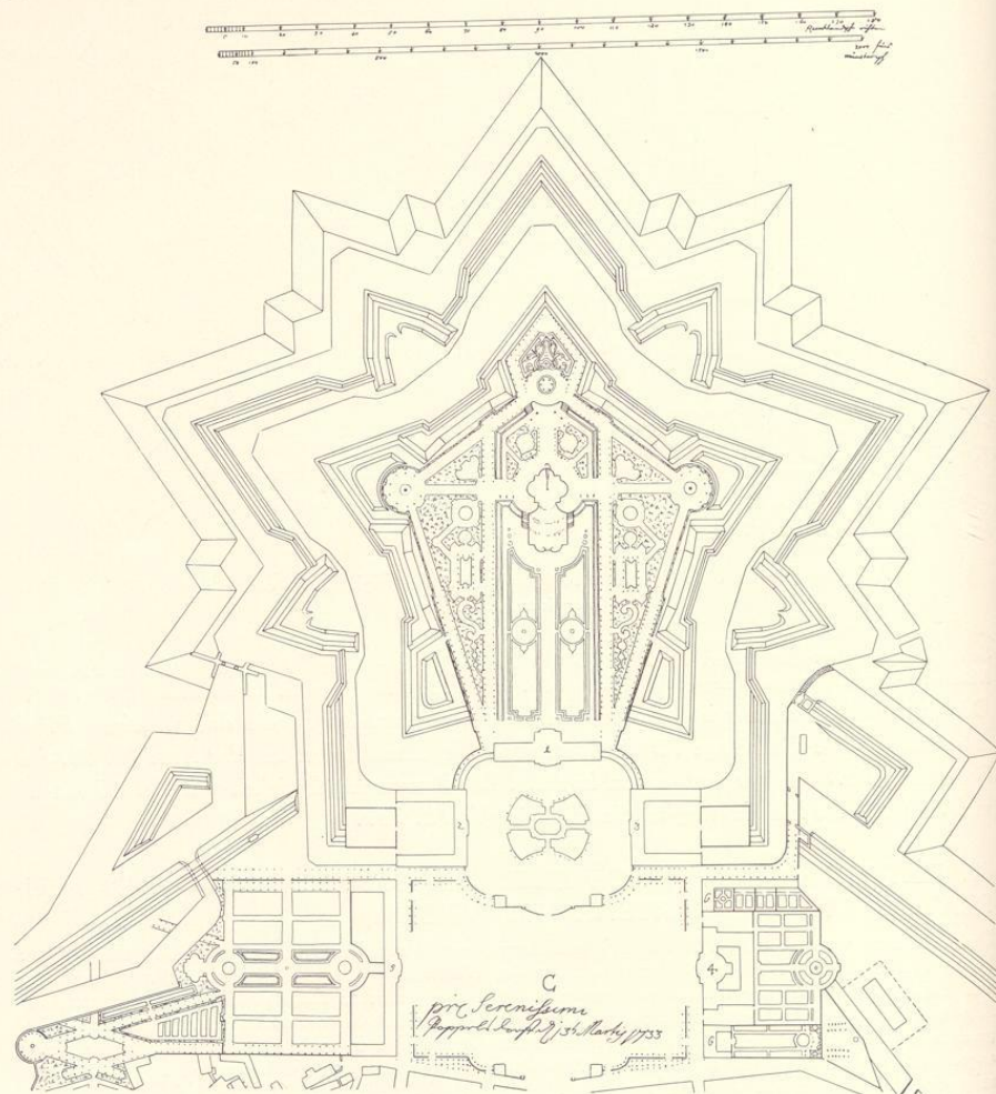
Abb. 39. Entwurf der Anlage eines Residenzschlosses, des Neuplatzes und des Hofgartens, 1733 (Verzeichnis Nr. 88, Pause)
