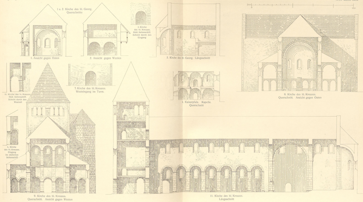
Stift. Kirche des hl. Georg. Kaiserpfalz. Aufgabe. Rekonstruktion
