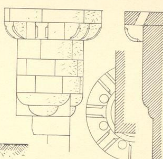
11-13. Eckerker am Turm
