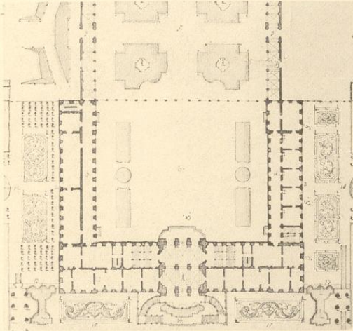
5. Entwurf von Kärcher (1. Vorschlag). Staatsarchiv Marburg
