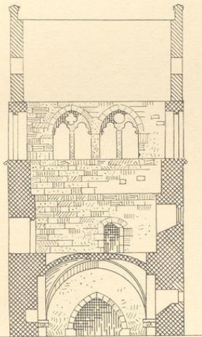
2. Turm. Längsschnitt
