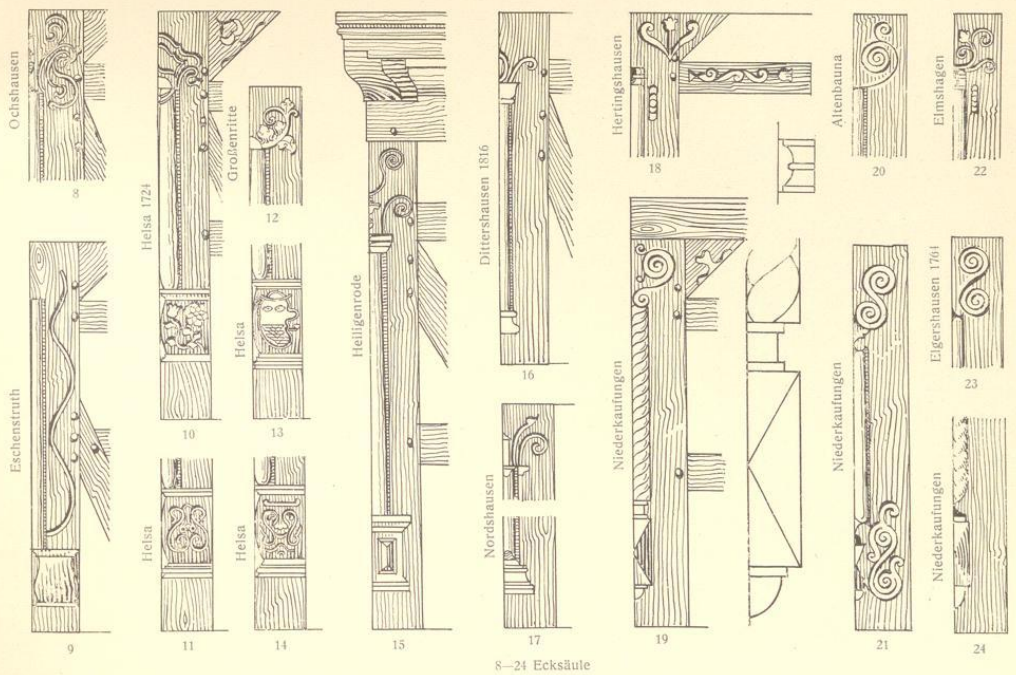
8-24 Ecksäule
