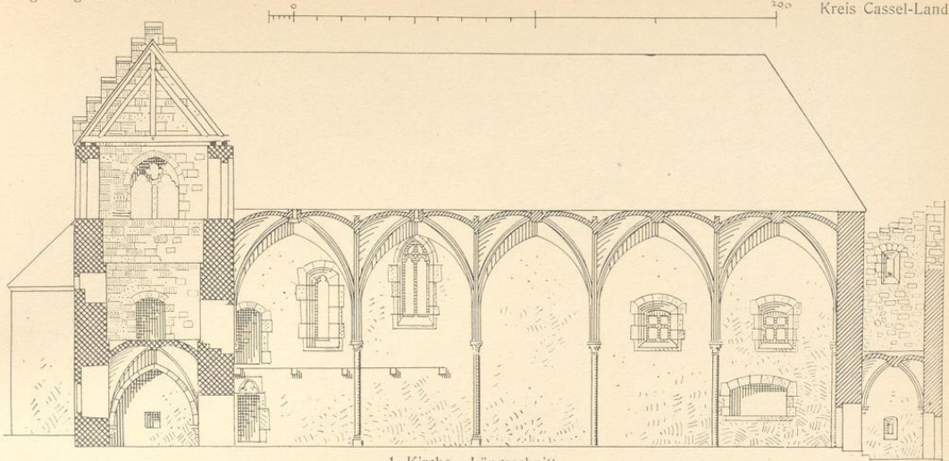
1. Kirche. Längsschnitt
