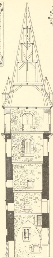
8. Turm. Querschnitt
