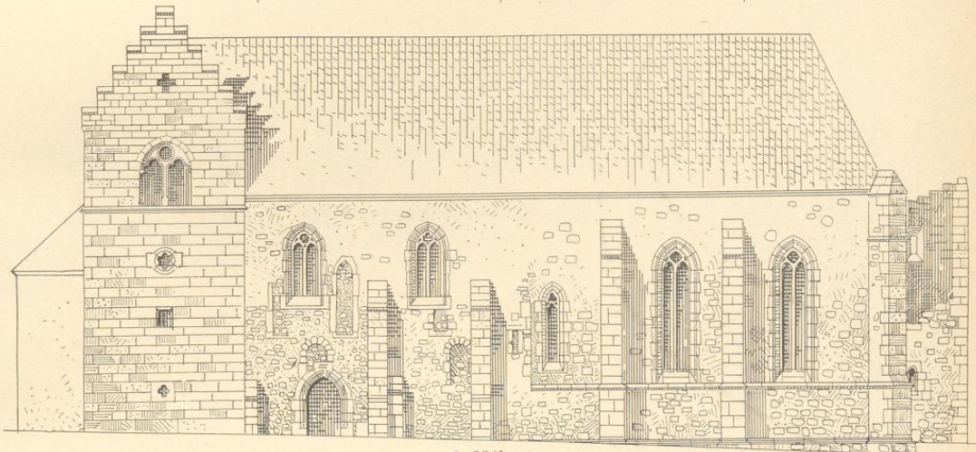
2. Südfront
