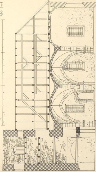
3. Schnitt, jetziger Zustand
