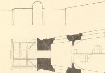
7. Hauptgesims des Helmes
