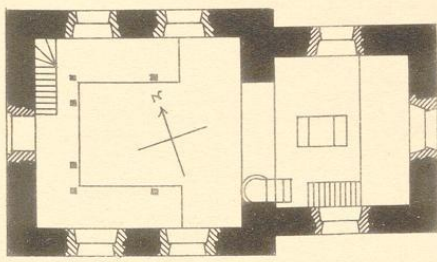
2. Grundriß
