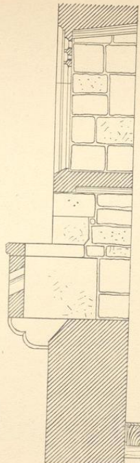
2. Schnitt
