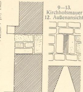
11. Schnitt
