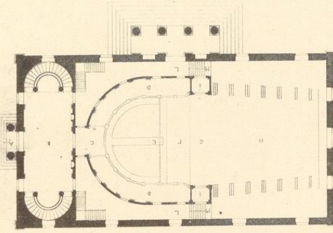
3. Grundriß. Früherer Zustand Zeichnung und Stich von L. Klenze
