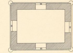
6. Turm. Grundriß der Glockenstube
