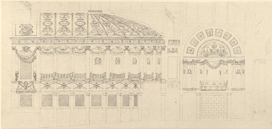
2. Längsschnitt. Zeichnung und Stich von L. Klenze
