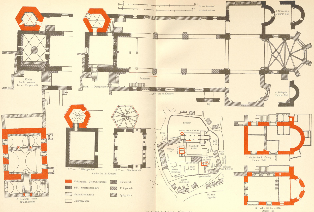
Stift. Kirche des hl. Georg. Kaiserpfalz Grundrisse. Jetztiger Zustand
