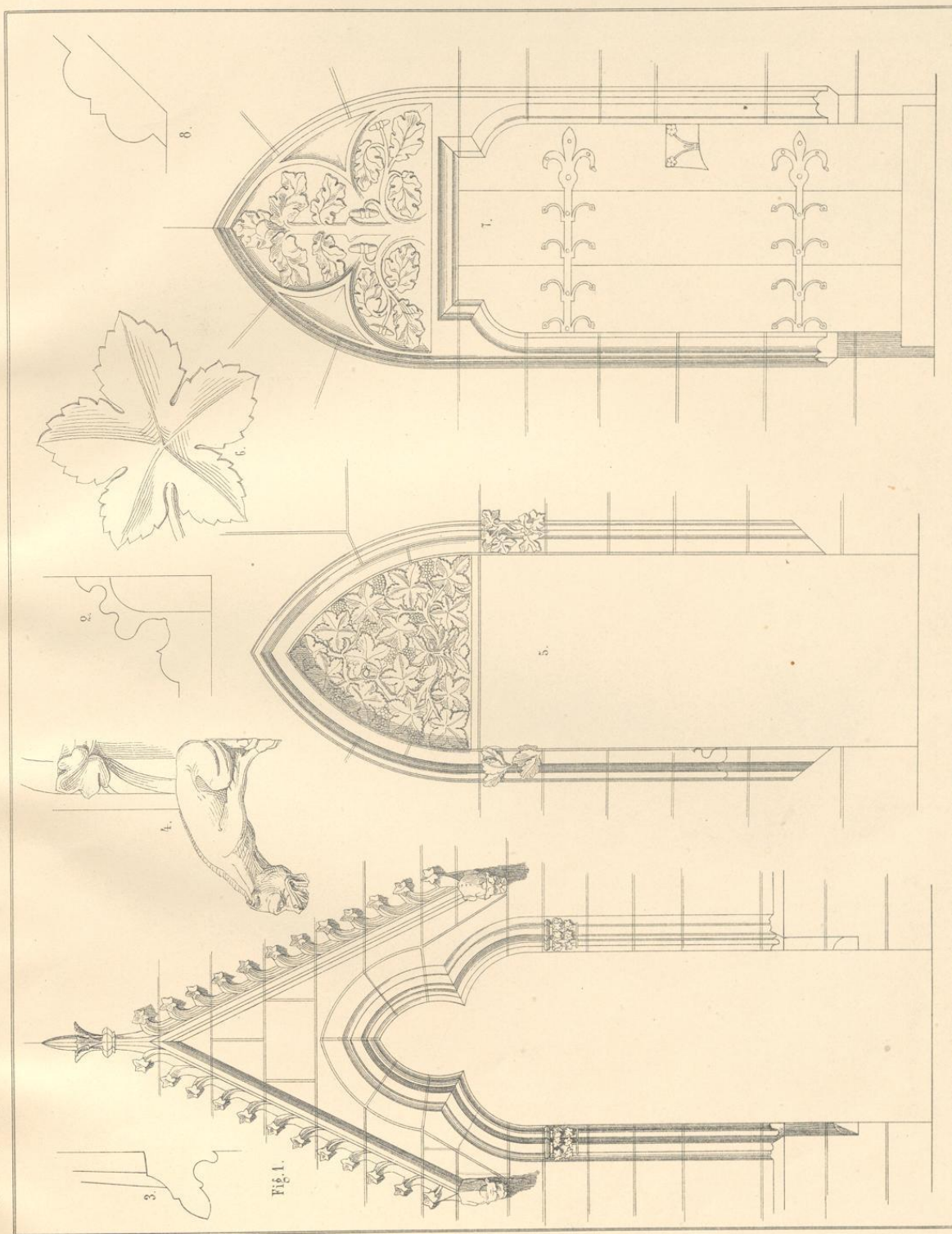
1-4 Südwestliche Pforte des Münsters zu Kölnar. — 5-6. Sächsischer Pforte zu Friedberg. — 7-8. Sächsischer Pforte zu Frankenberg.
