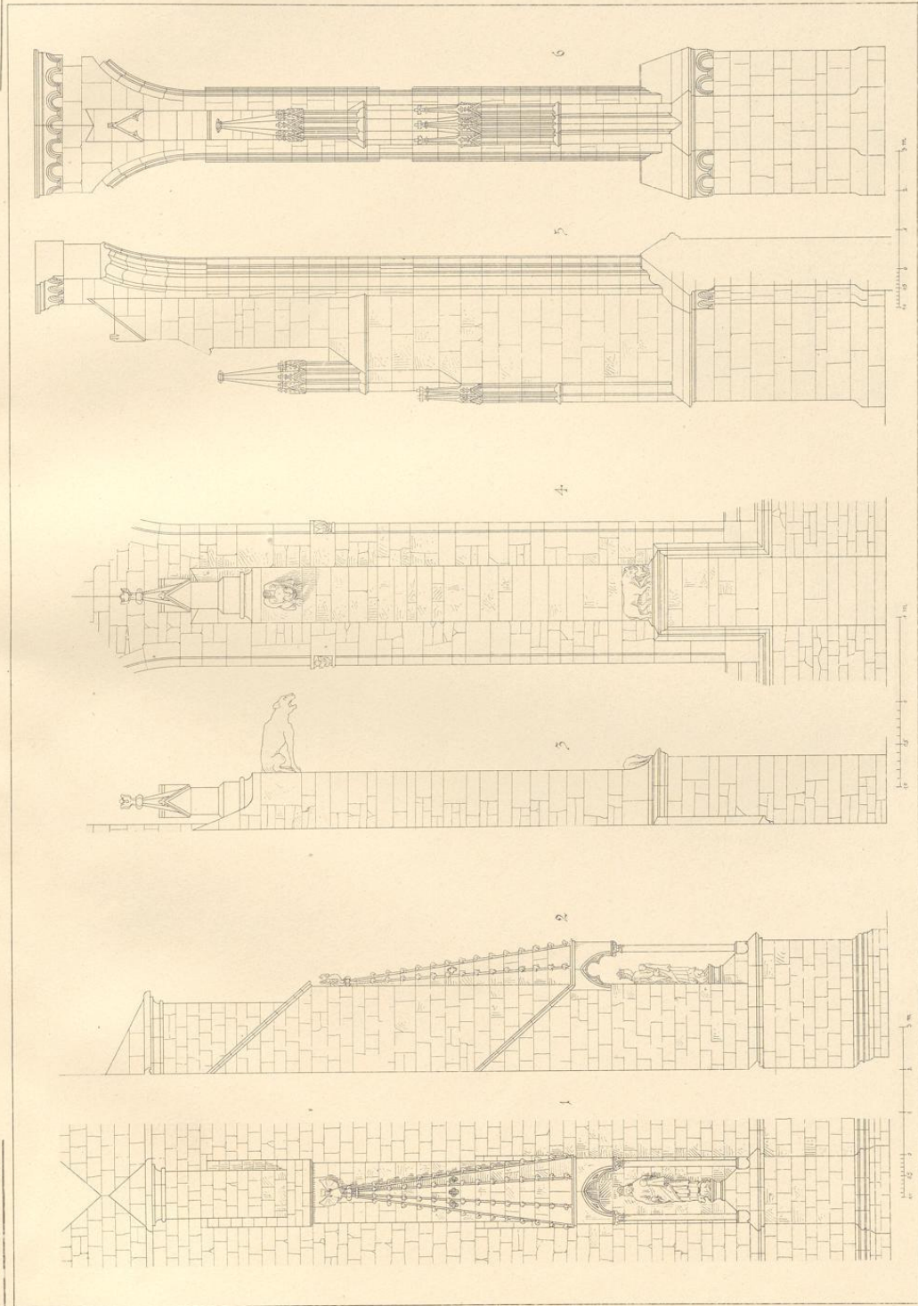
1—2. Strebepfeiler vom Dom in Minden. — 3—4. Chorstrebepfeiler von der Marienkirche in Lemgo. — 5—6. Chorstrebepfeiler aus Walfenried.
