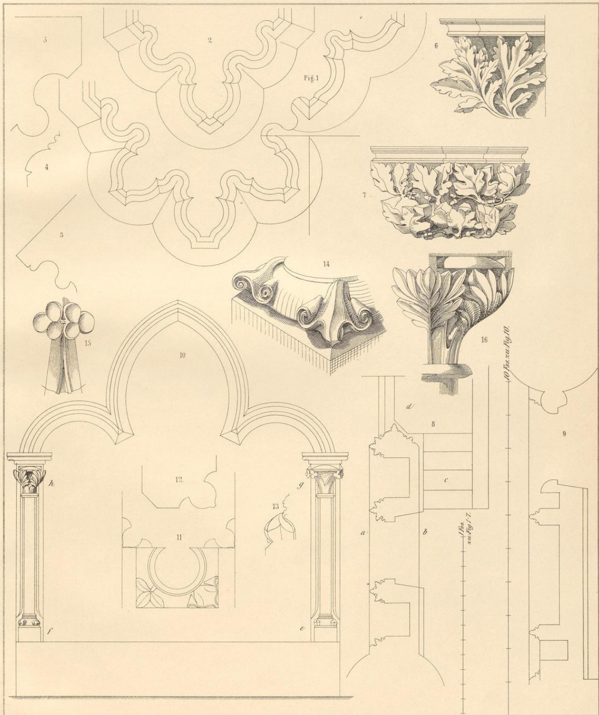
1—9. Chorjranken aus Haina (vgl. Taf. 87). 10—16. Wandstuh aus Mühlhausen in Thüringen.
