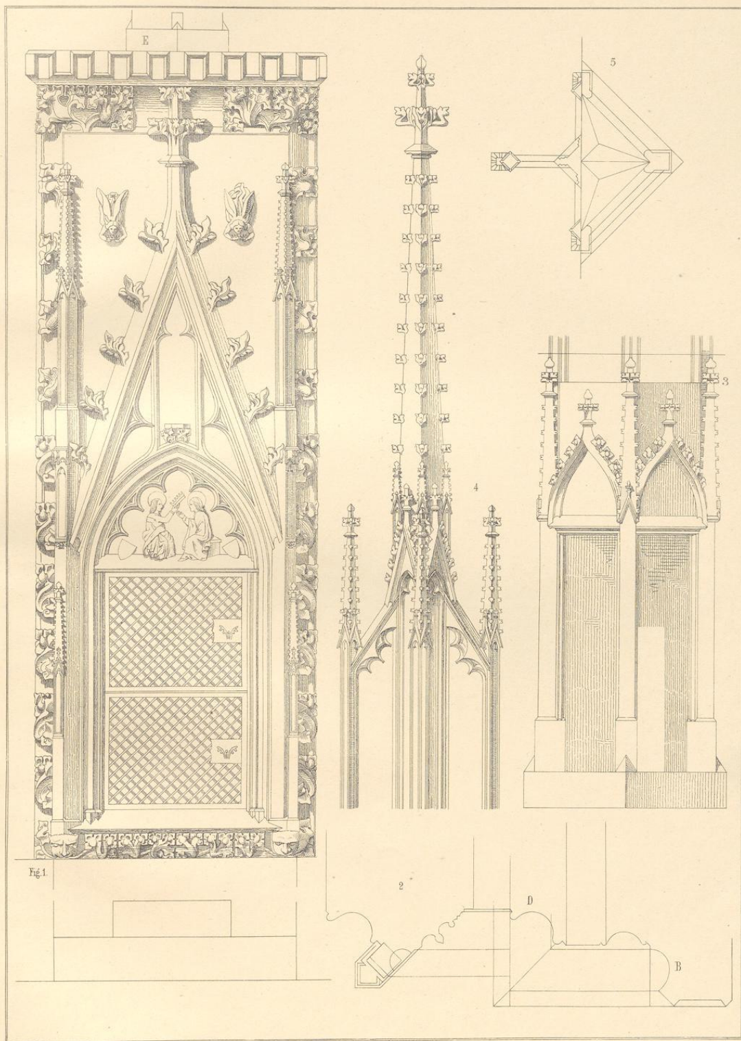
Tabernakel aus Gelnhausen.
