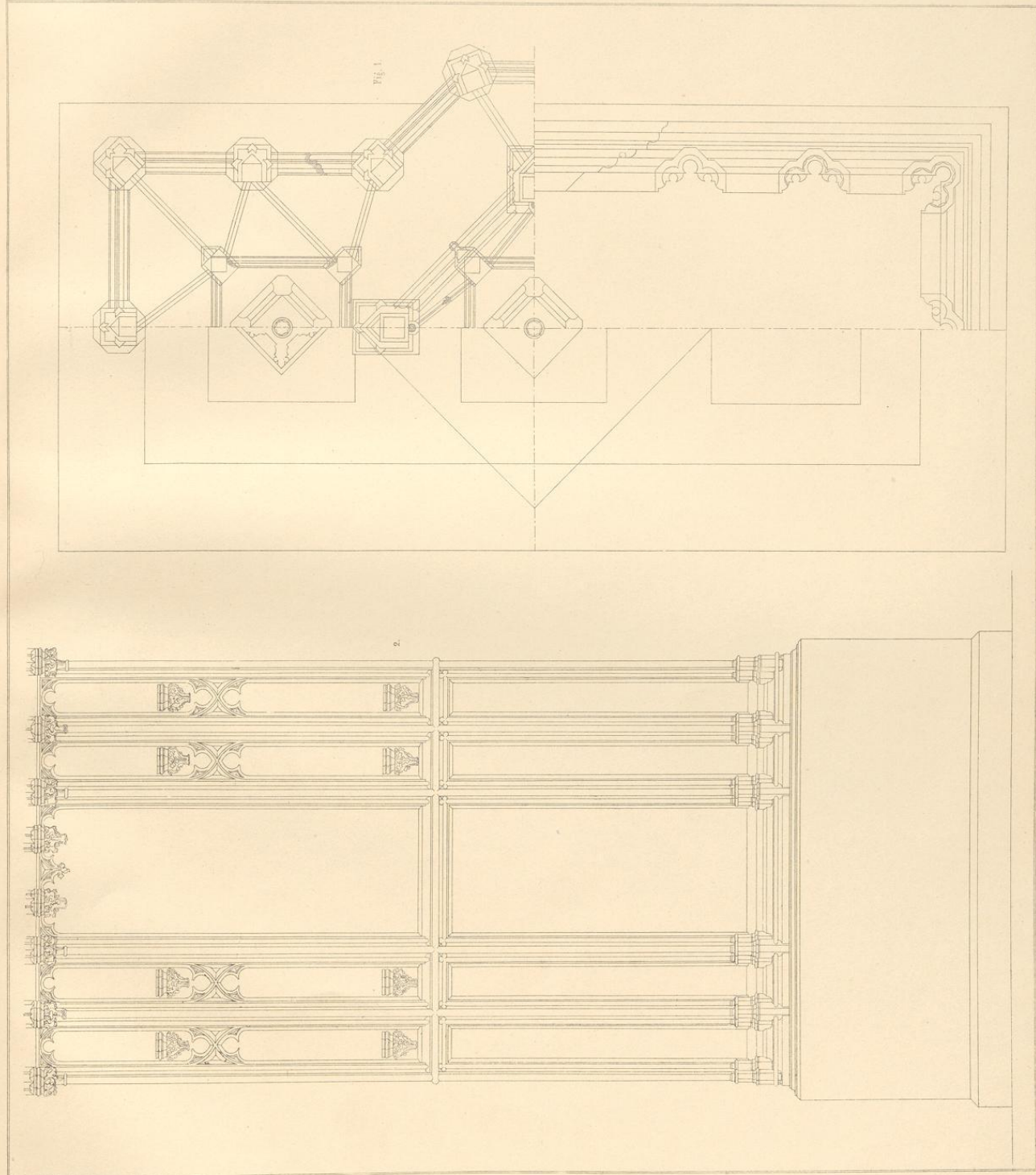
Stuhlgang aus der Marienkirche in Soest (vgl. Taf. 80).
