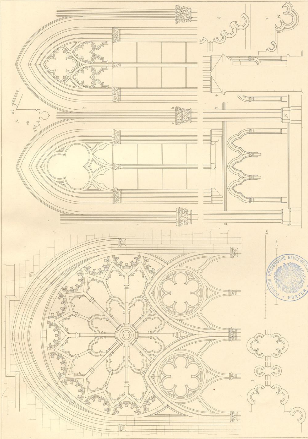
1—2. Fenster vom Dom in Minden. — 5—7. Chorfenster der Martinikirche in Minden.
