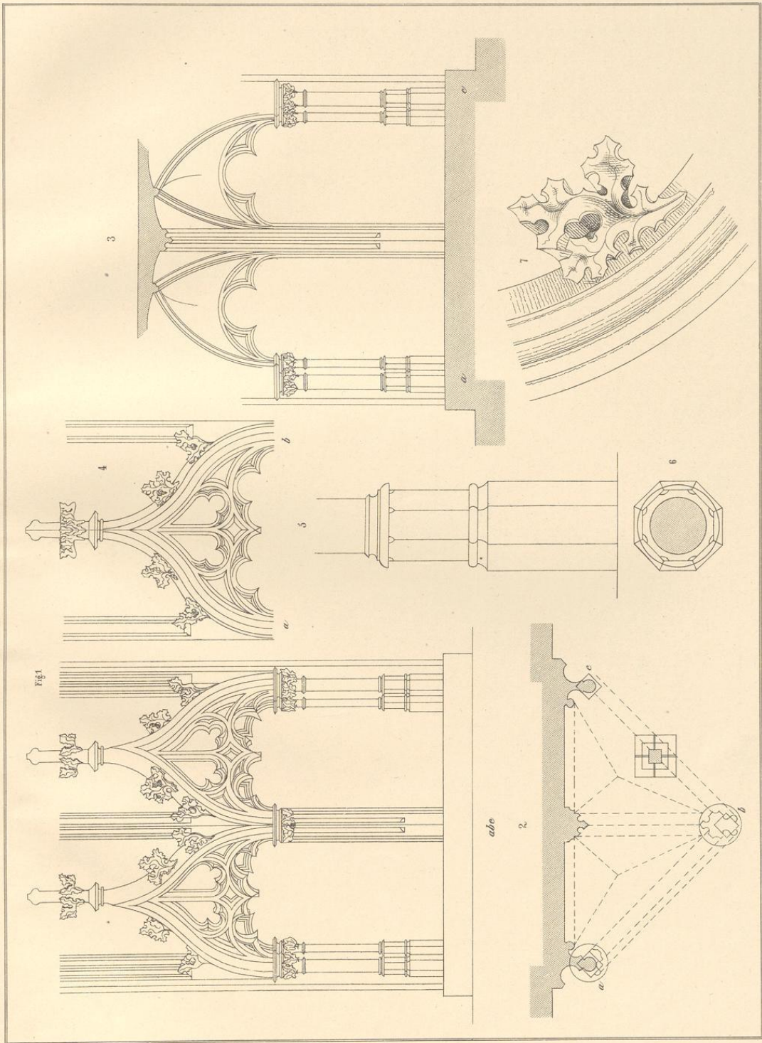
Unterbau eines Tabernakels aus Kirchhoven.
