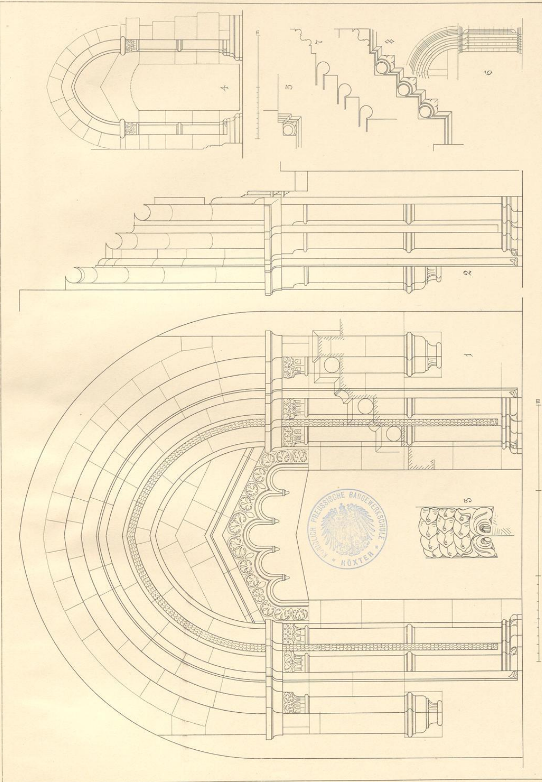
1—3. Portal aus Wieprechtshausen. — 4—5. Pforte aus Wieprechtshausen. — 6—8. Portal vom jüd. Querschiff des Domes in Minden.
