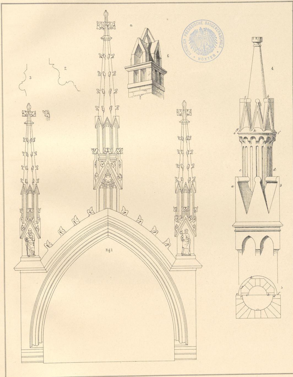
1—3. Mauerblende aus der Stadtkirche in Warburg. — 4—5. Siebelfürmchen aus Straßburg (vgl. Taf. 52). — 6. Schornstein aus Besançon.
