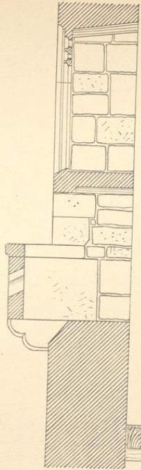
2. Schnitt
