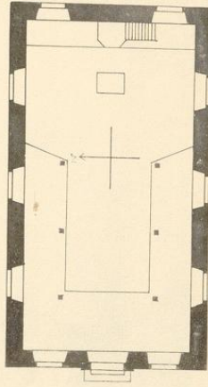
6. Grundriß
