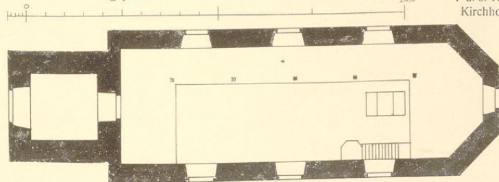
9. Grundriß
