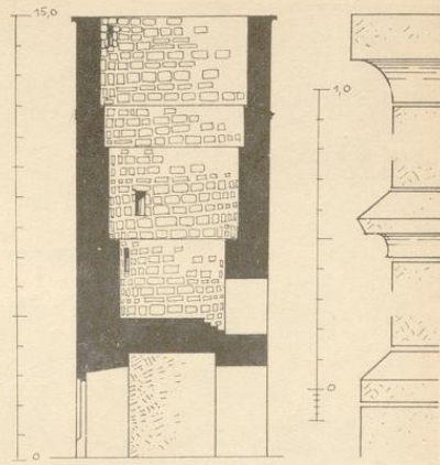
2. Turm. Schnitt
