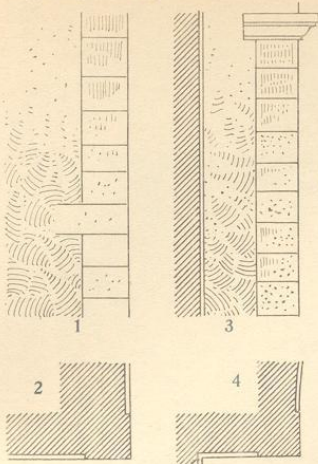
1—4. Eckfassung der Putzflächen im Äußeren im Inneren in der Kirche des hl. Georg
