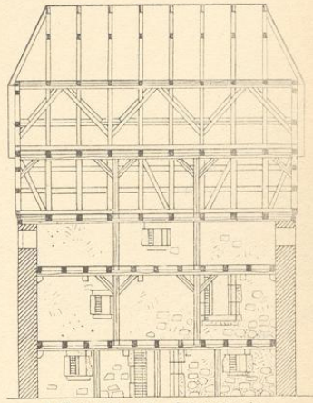
4. Zehntscheuer. Längsschnitt
