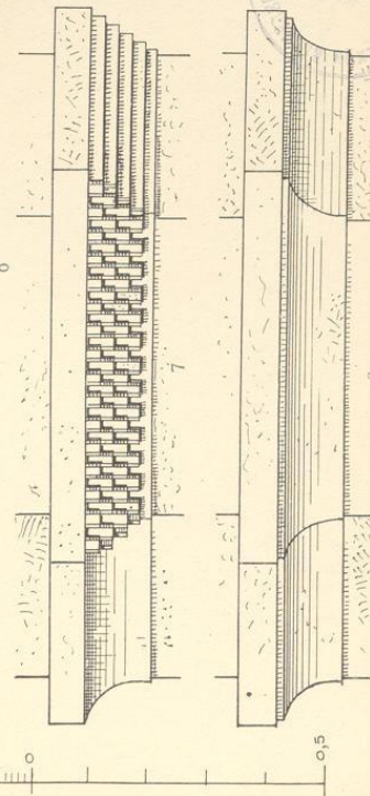
6-8. Gewölbekämpfer
