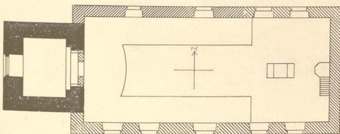
10. Grundriß
