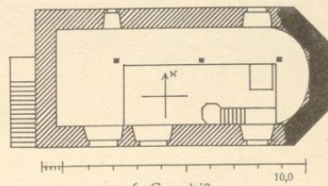
6. Grundriß
