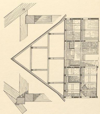
6. Querschnitt
