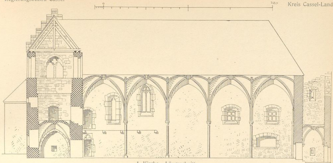
1. Kirche. Längsschnitt
