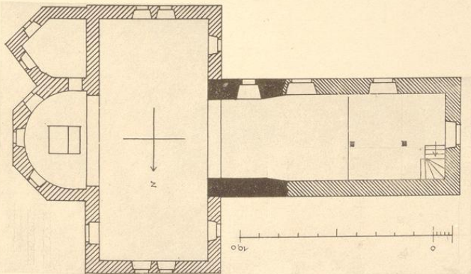
1. Grundriß
