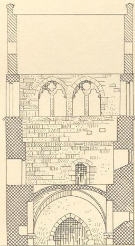
2. Turm. Längsschnitt
