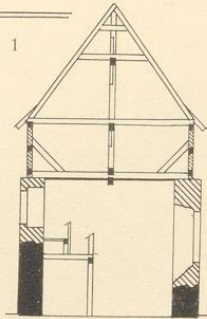
6. Schnitt
