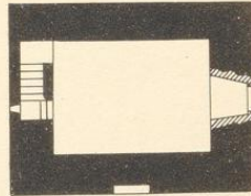
7. Turm. Grundriß des Erdgeschosses in Höhe der Treppe geschnitten
