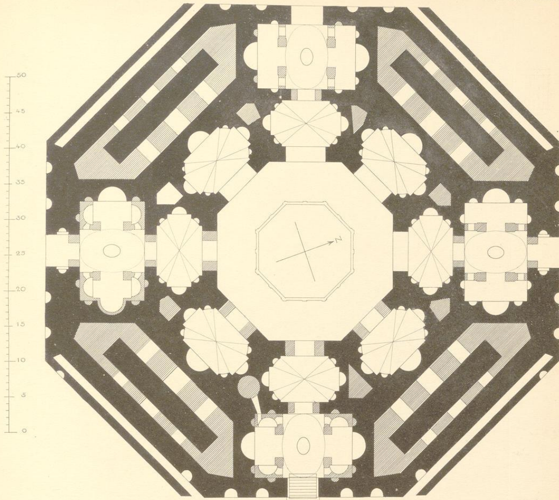
1. Grundriß des Erdgeschosses
