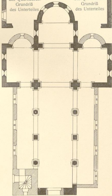
5. Grundriß. Jetziger Zustand
