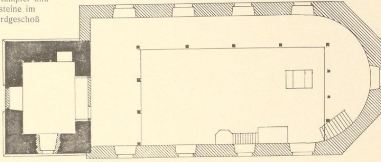
11. Grundriß
