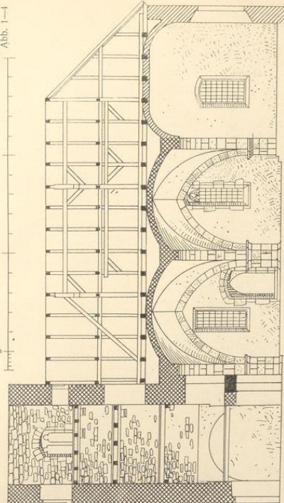
3. Schnitt, jetziger Zustand
