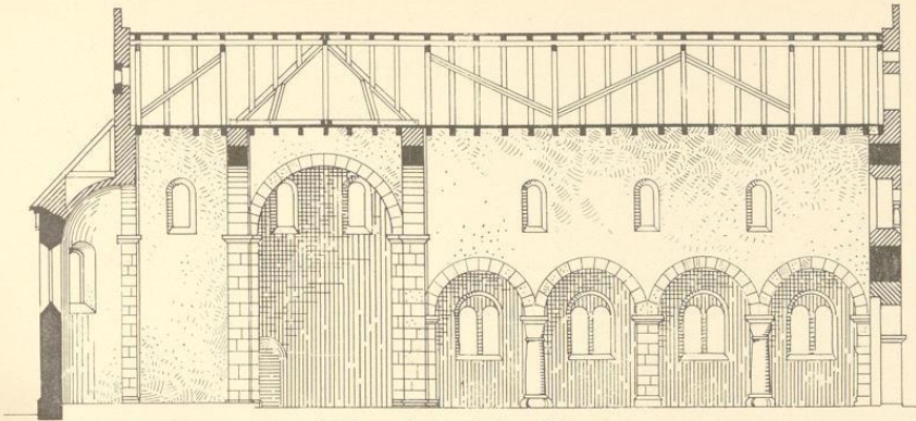
1. Längsschnitt. Jetziger Zustand
