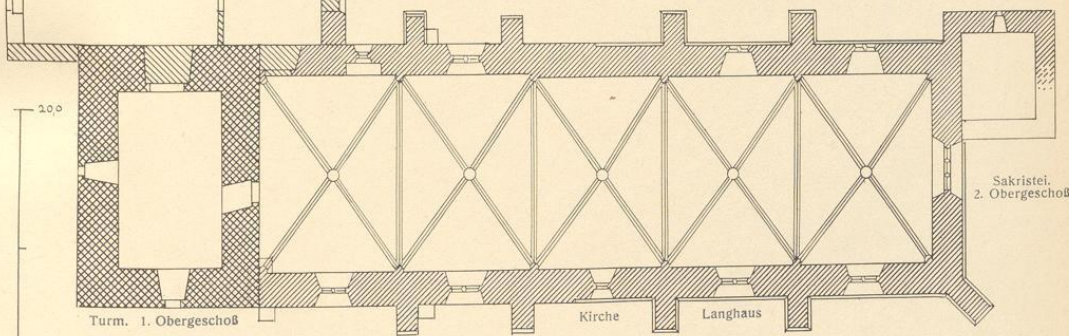
2. Kirche und Klausur. Grundriß. Jetziger Zustand
