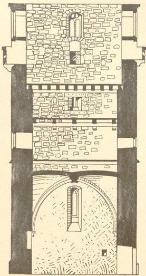
5. Turm. Schnitt von Nord nach Süd
