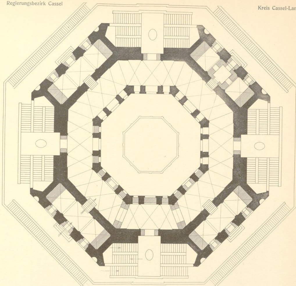
1. Grundriß des Zwischenstockes
