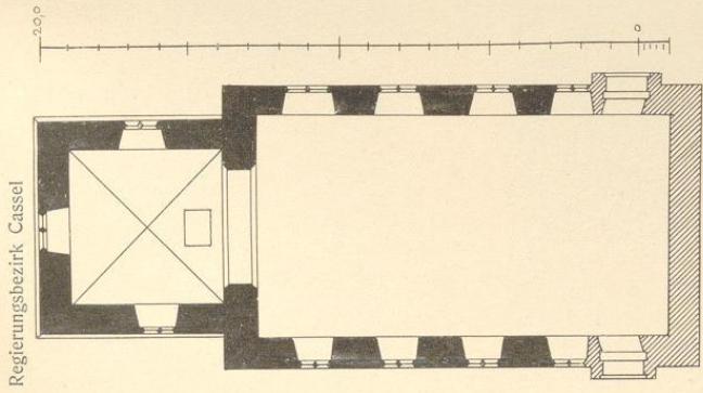
1. Grundriß
