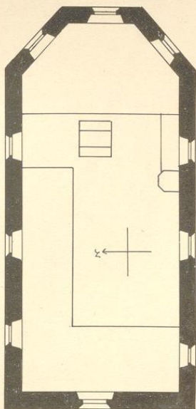
2. Grundriß
