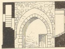
10. Turm. Längsschnitt durch das Erdgeschoß
