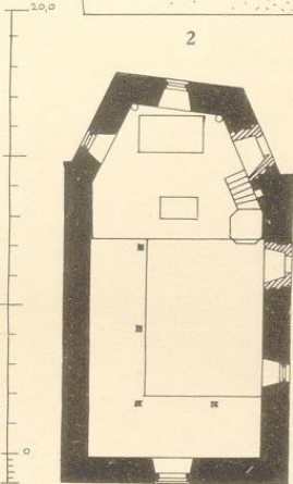
5. Grundriß
