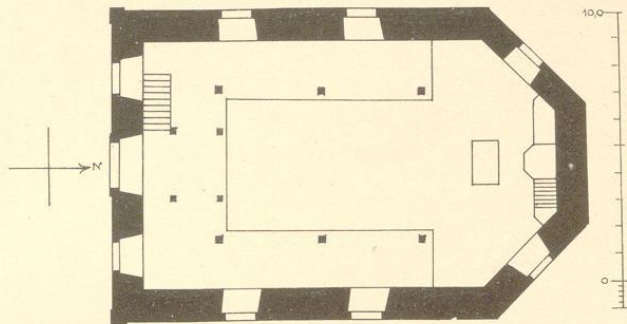
2. Grundriß
