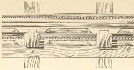
1. Crumbach Quergebälk
