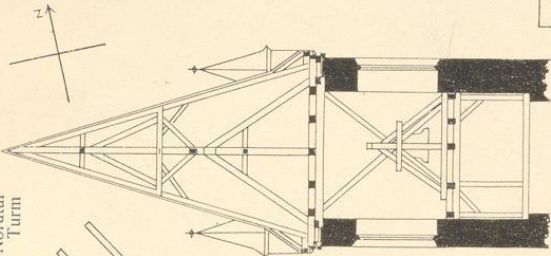
5. Grundriß. Rekonstruktion
