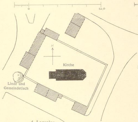
4. Lageplan
