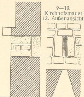
11. Schnitt
