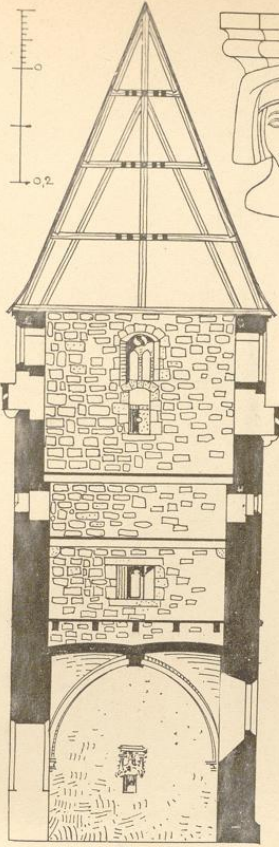
4. Turm. Schnitt von West nach Ost
