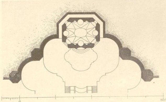
4. Grundriß. Entwurf. Rekonstruktion
