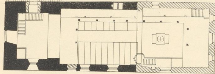
6. Grundriß. Jetztiger Zustand
