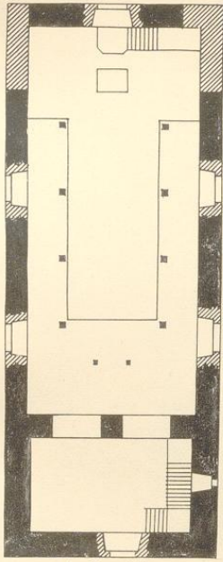
1. Grundriß. Jetziger Zustand
