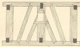
7 u. 8. Glockenstuhl
