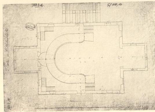
2. Grundriß. Entwurf. Murhardbibliothek Cassel
