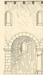
2. System des Langhauses. Rekonstruktion
