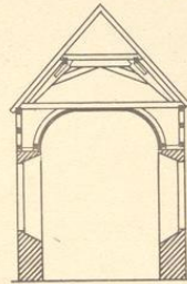
7. Schnitt
