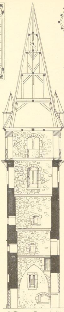
8. Turm. Querschnitt
