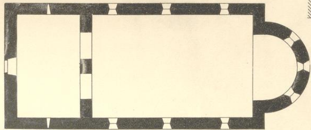
2. Grundriß Rekonstruktion
