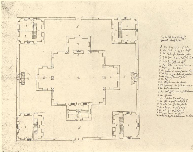
3. Grundriß. Entwurf
