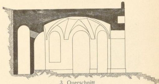
3. Querschnitt
