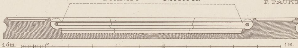
SCHNITT NACH A.
