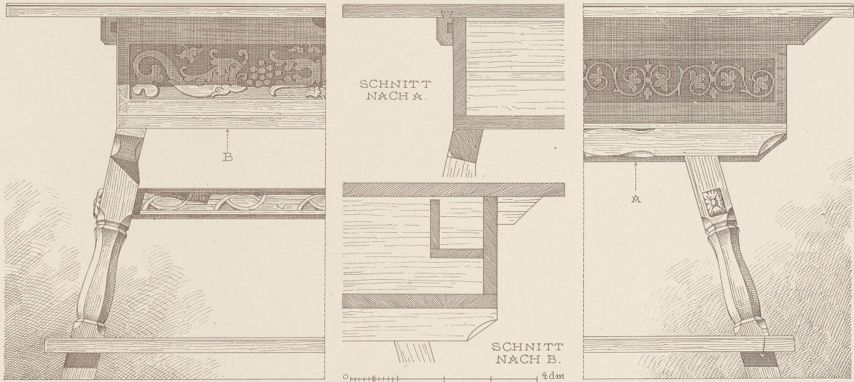
A.B. TISCH AUS DER VORBILDER-SAMMLUNG DER K.K. FACHSCHULE FÜR HOLZINDUSTRIE.
