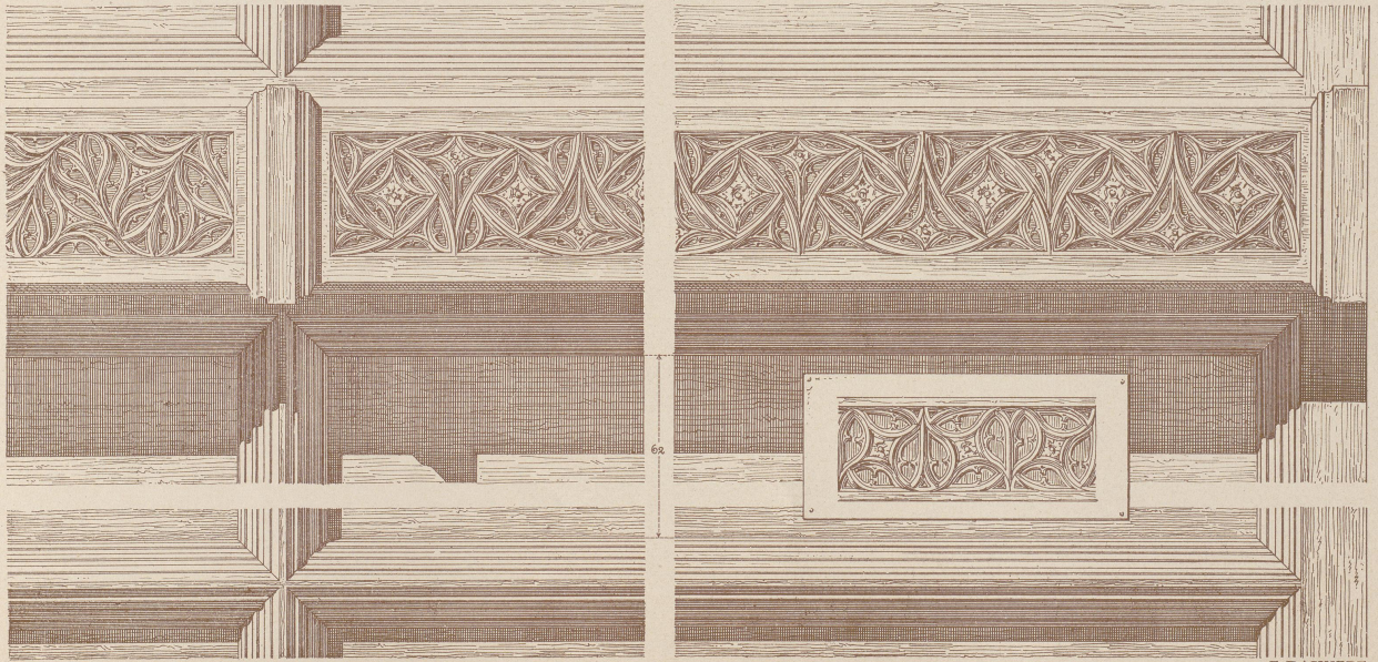
SYSTEM EINER HOLZDECKE IM ANSITZE WEGGENSTEIN.
