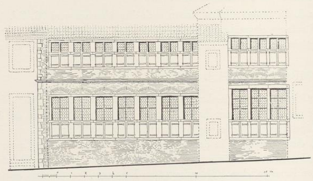
Abb. 968. Rekonstruktion der Südseite des Renaissance-Hauses Maßstab 1 : 200
