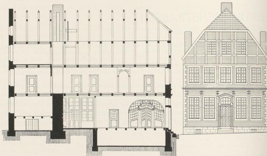
Abb. 1016. Längsschnitt des Hauses Rosenplatz 11. Maßstab 1 : 200
