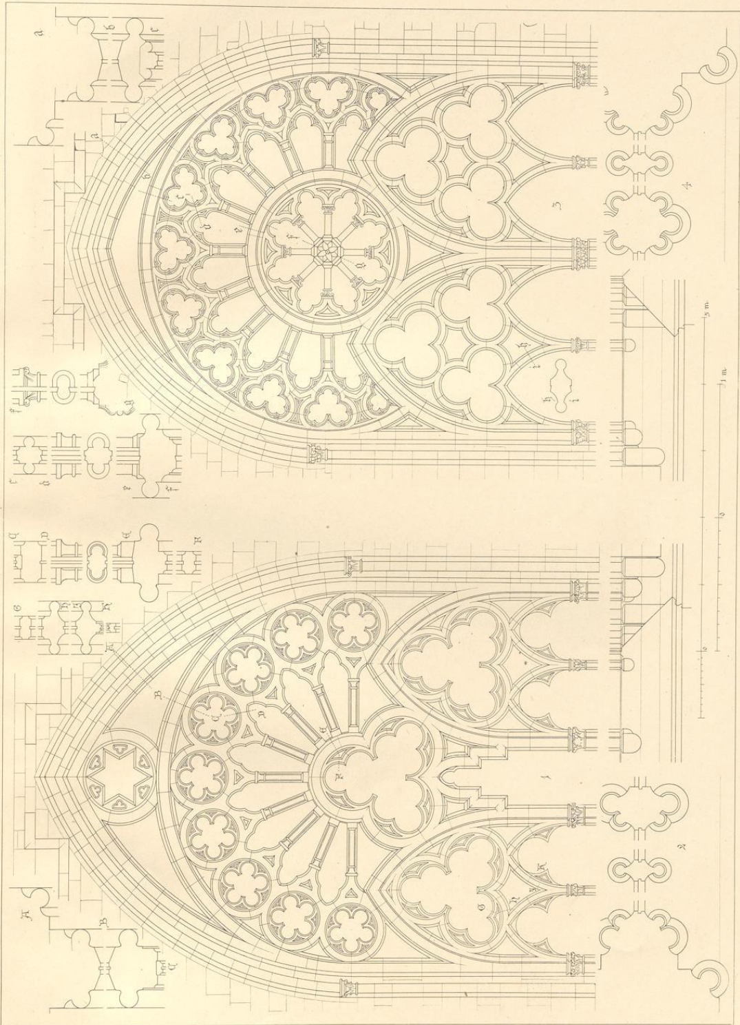
fenster vom Dom in Minden.
