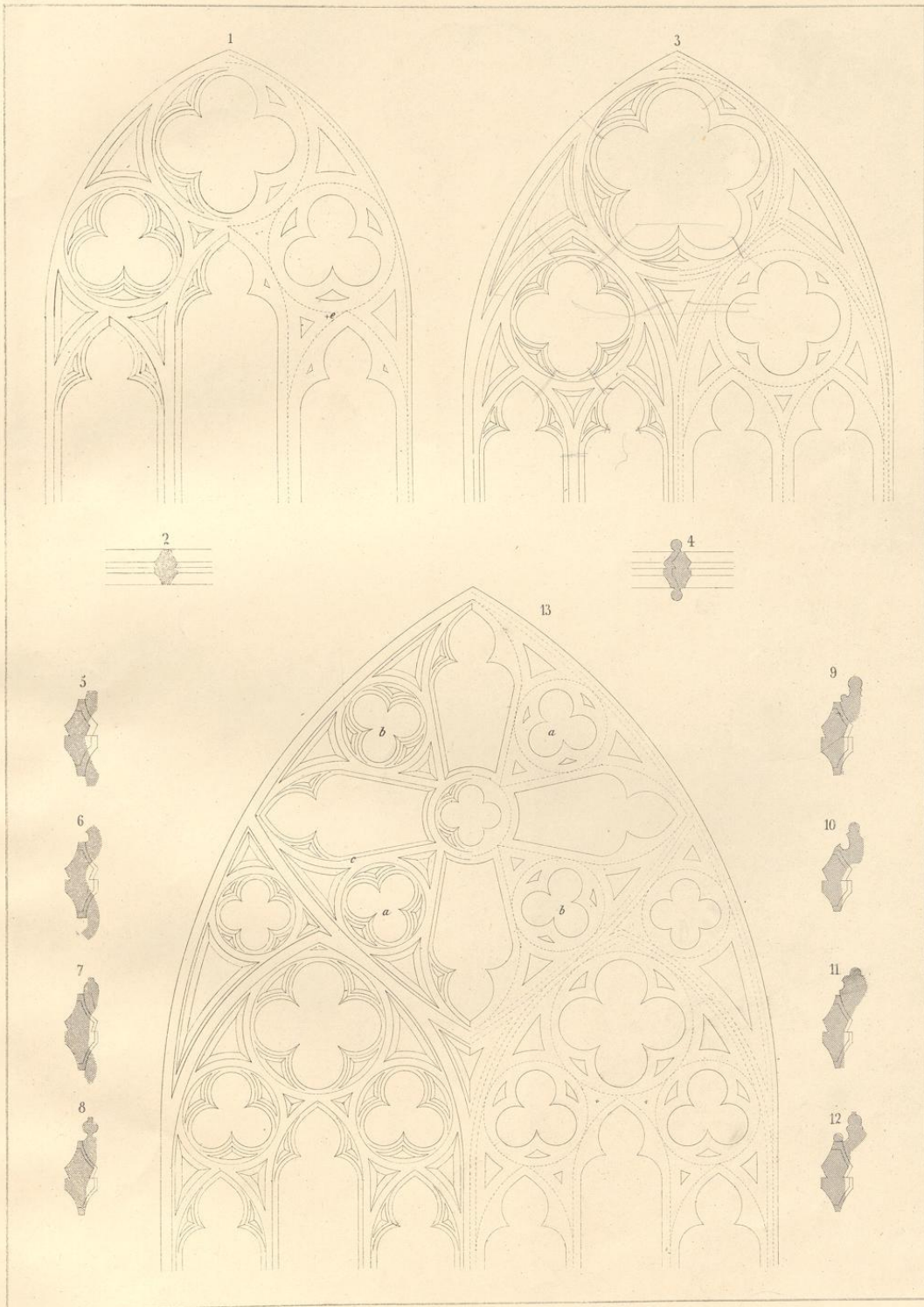
Fenstermaßwerke.
