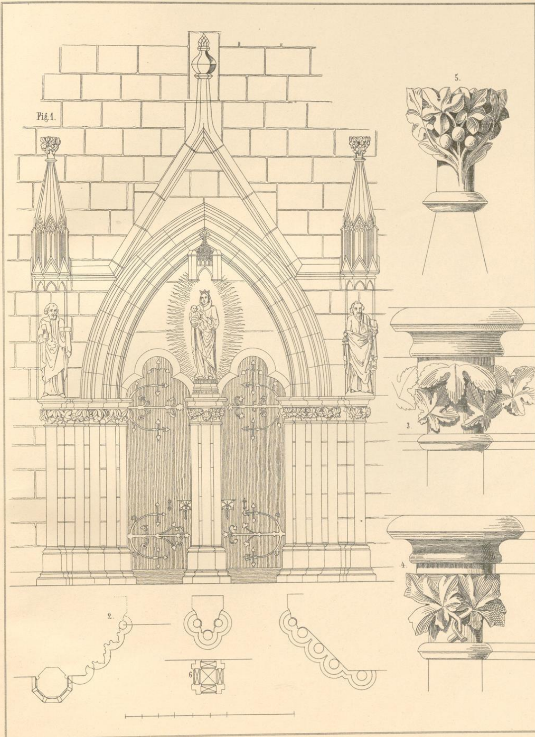
Portal der Kirche zu Volkmarfen.
