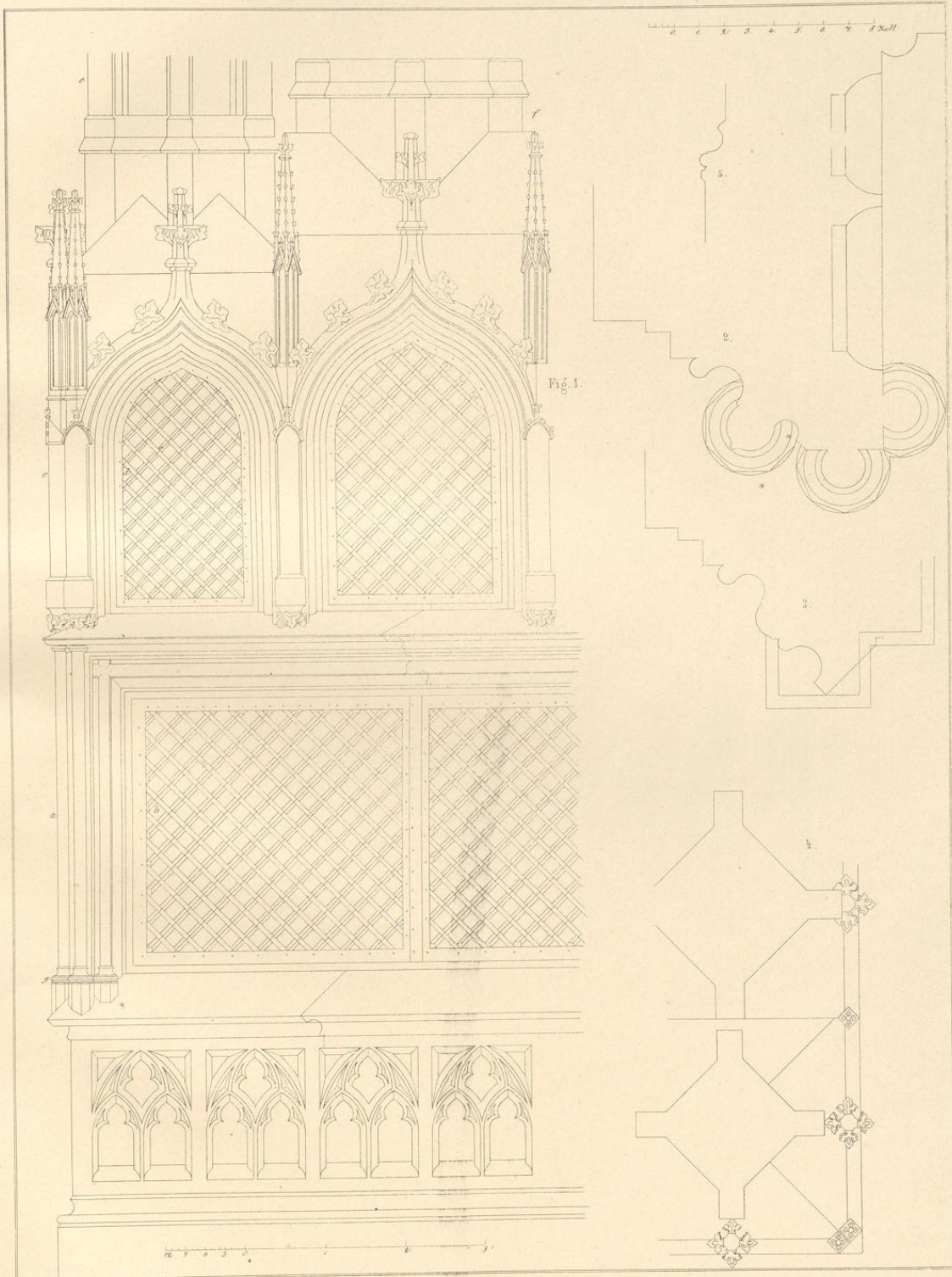
Tabernakel aus Dortmund (vgl. Taf. 69, Fig. 1 und 2).
