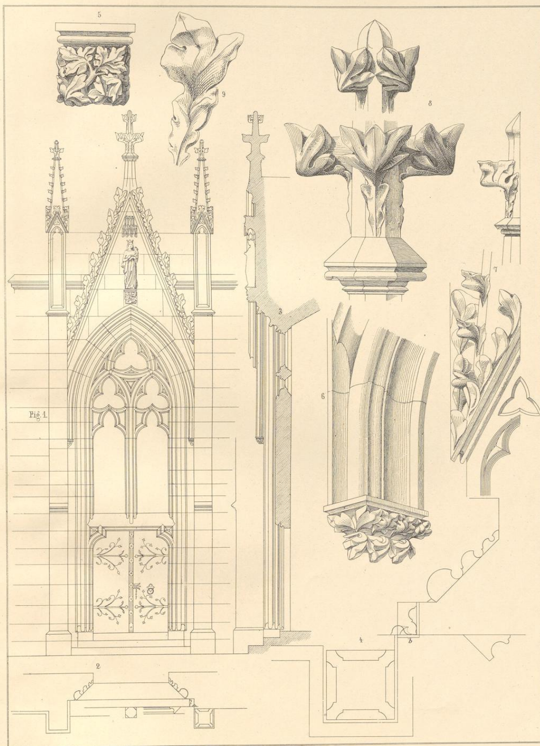
Thür der Kirche zu Haina.
