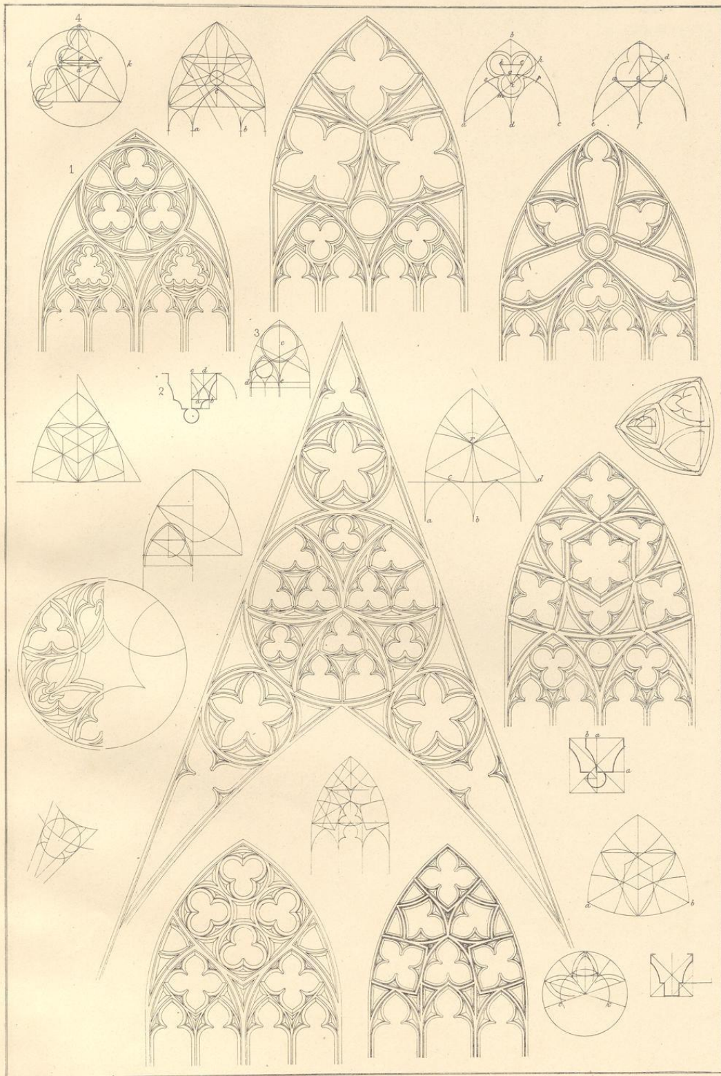
Maßwerke aus Erfurt, Ulm und anderen Orten.
