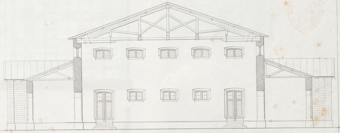
Durchschnitt nach A. B.
