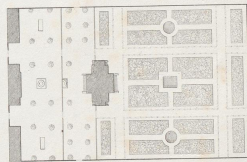
Grundriss des Erdgeschosses
