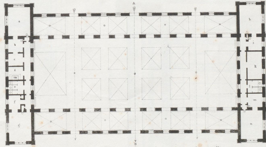
Schranngעהäude.
