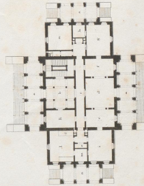
Grundriss des 1. Obergeschosses
