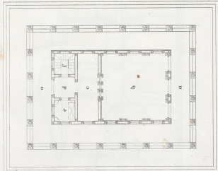
Grundriss
