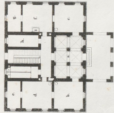
B. Grundriss der unteren Kirche
