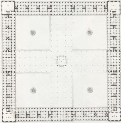
3. Grundriss der oberen Etage.
