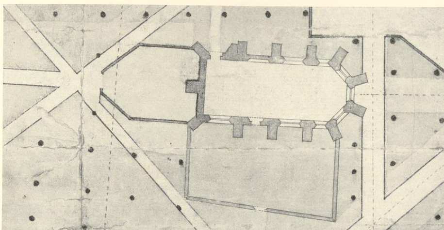
Abb. 2021. Grundriß der Jakobikirche Aufmessung von J. C. Schlaun, 1748
