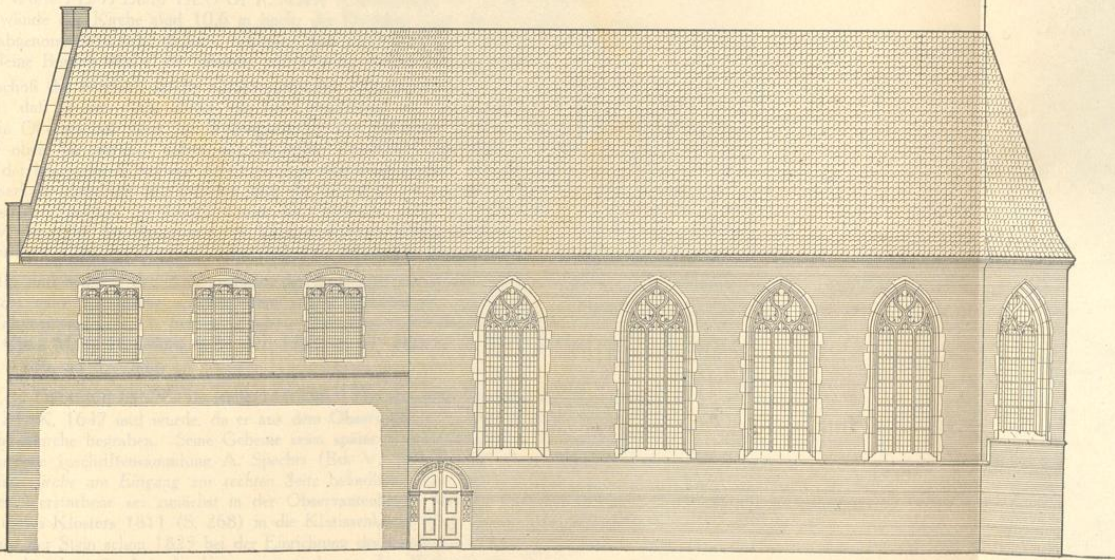
Abb. 2068. Aufriß der Westseite der Klarissenkirche an der Stubengasse
