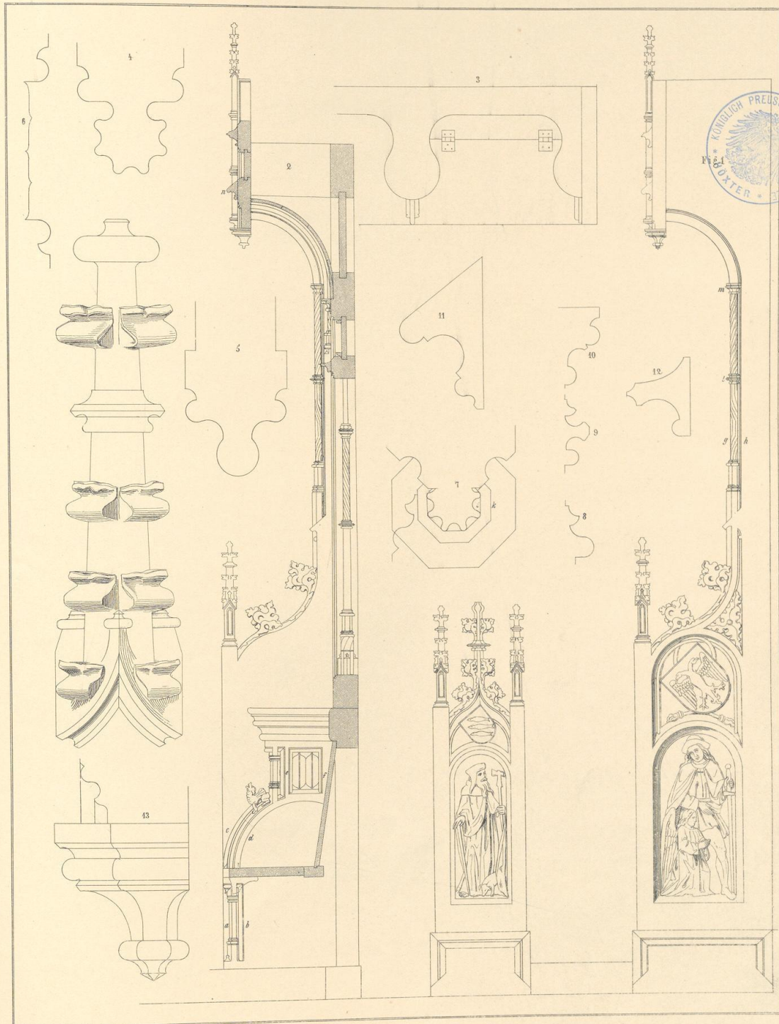
Gestühl in der St. Marienkirche zu Lübeck.
