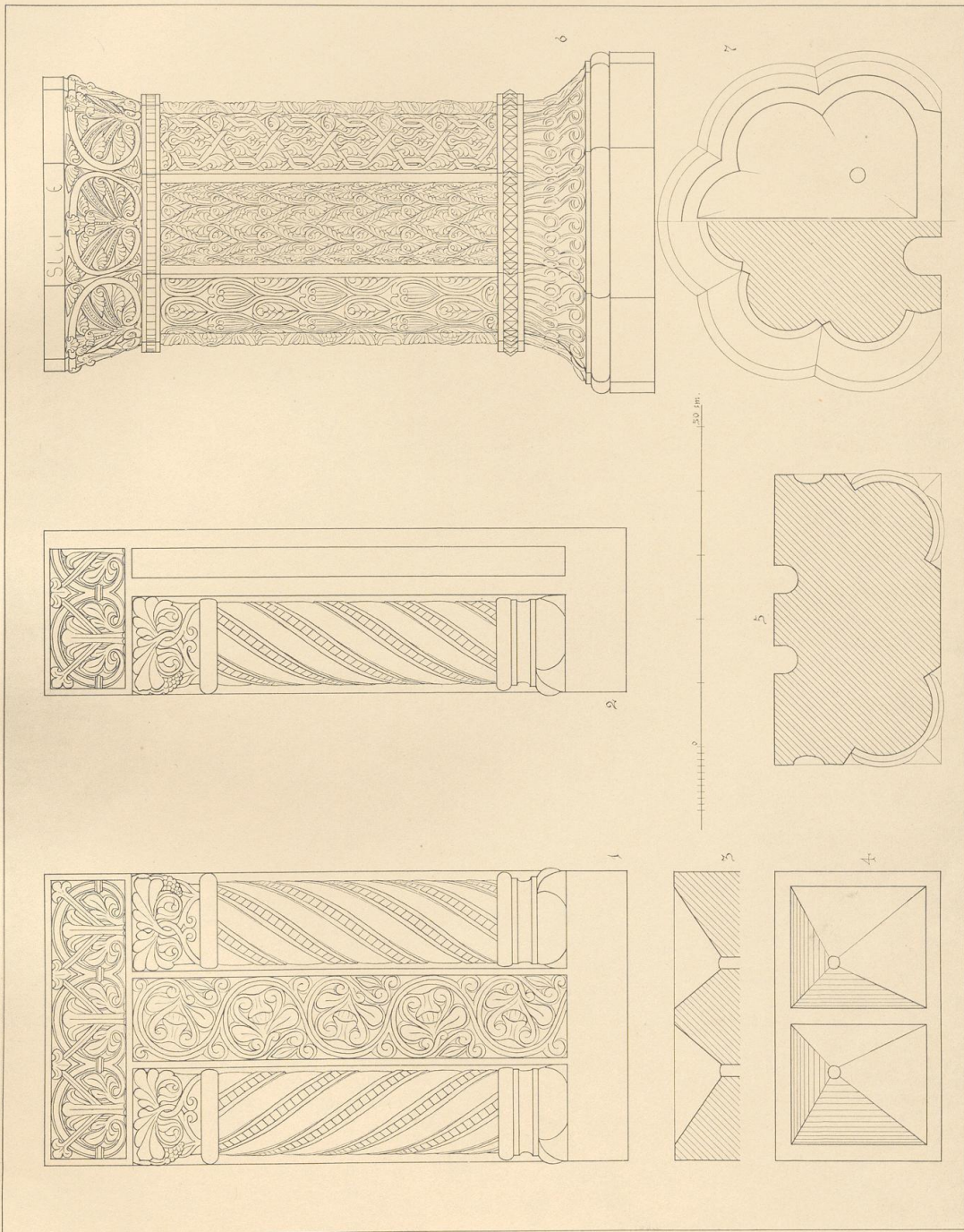
Piscinen aus Amelunghorn.
