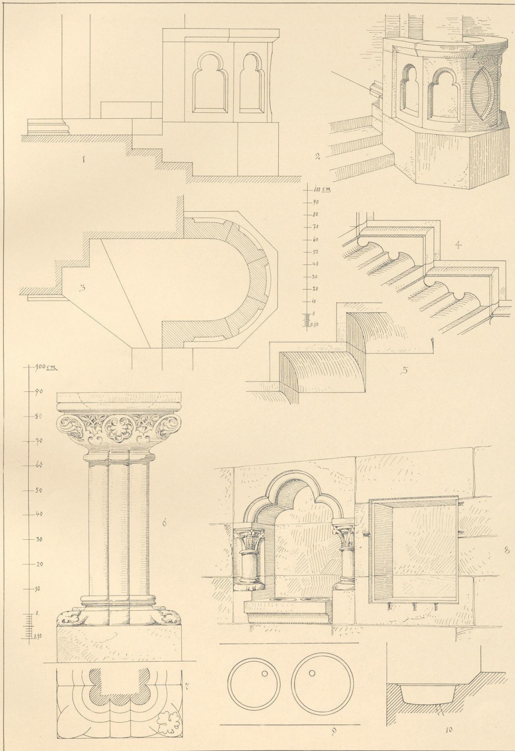
1—5. Kanzel zu Wieprechtshausen. 4—5. Kanzeltreppen aus Mühlhausen und Ouderstadt. 6—8. Piscinen aus Walkenried. 9—10. Piscina aus Riddagshausen.
