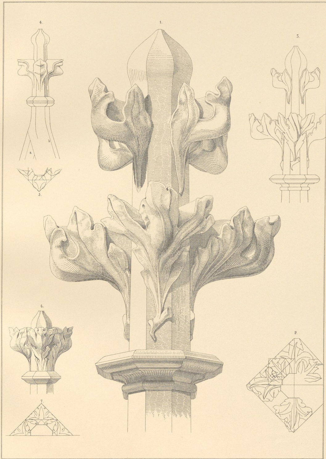
1—3. Kreuzblume aus dem Dome in Regensburg. 4—5. Kreuzblume aus der Wiefentirche in Soest. 6—7. Kreuzblume von einem Tabernakel in Grebenstein.
