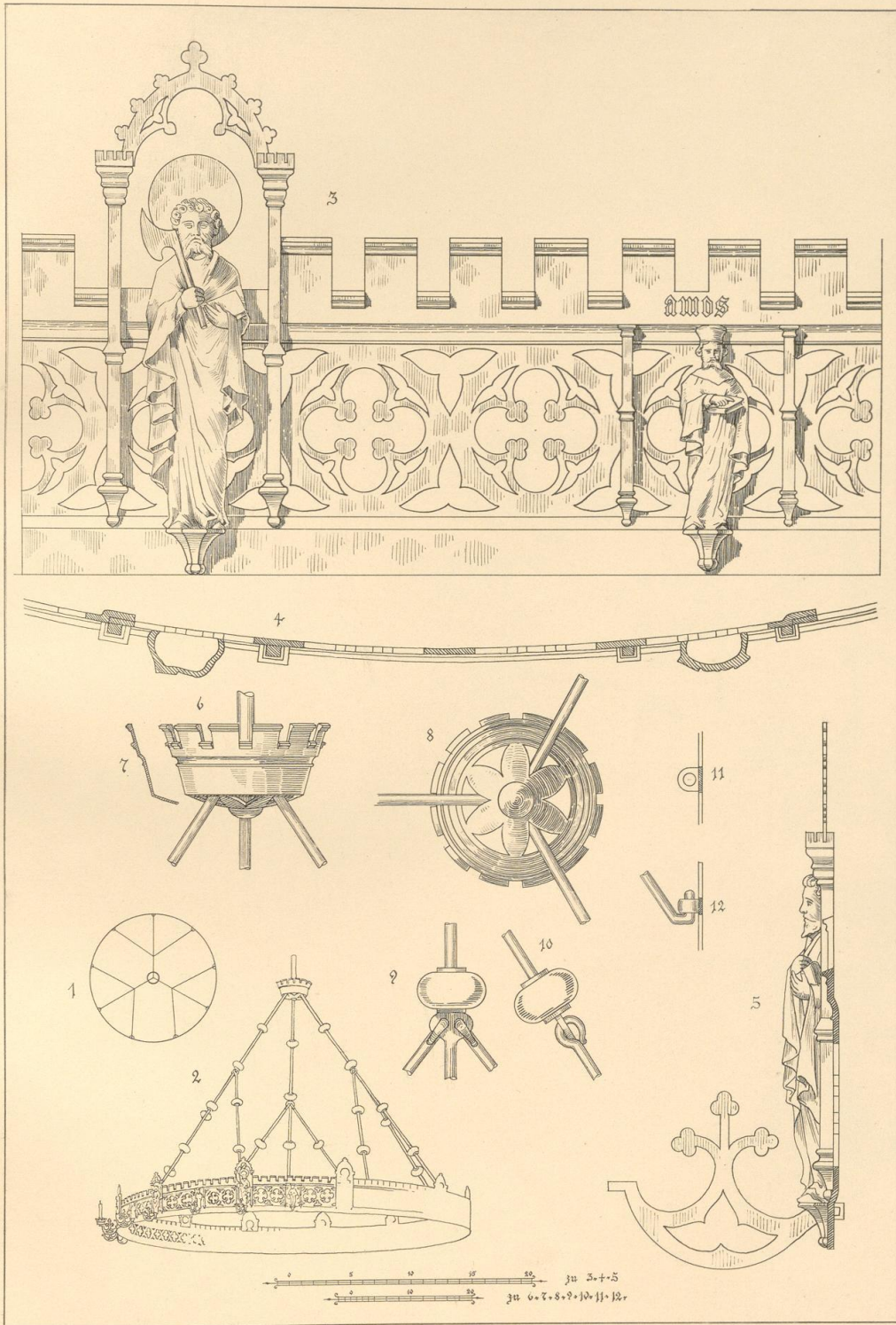
Radleuchter aus der Megandirkirche in Einbeck.
