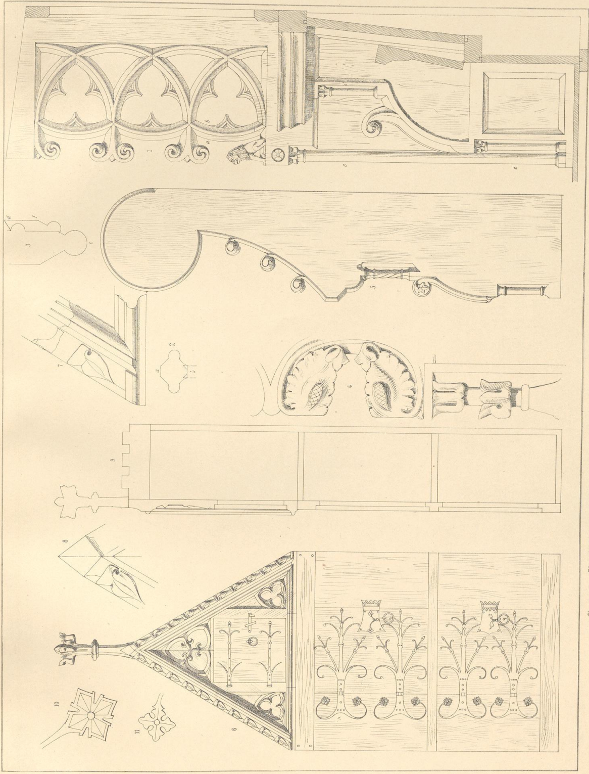
Fig. 1—3. Chorgestühl aus Friedberg. Fig. 4. Einzelheit zu Tafel 119. Fig. 5. Seitenwand eines Geyhüles aus der Predigerkirche in Erfurt. Fig. 6—11. Schrein aus Gelnhausen.
