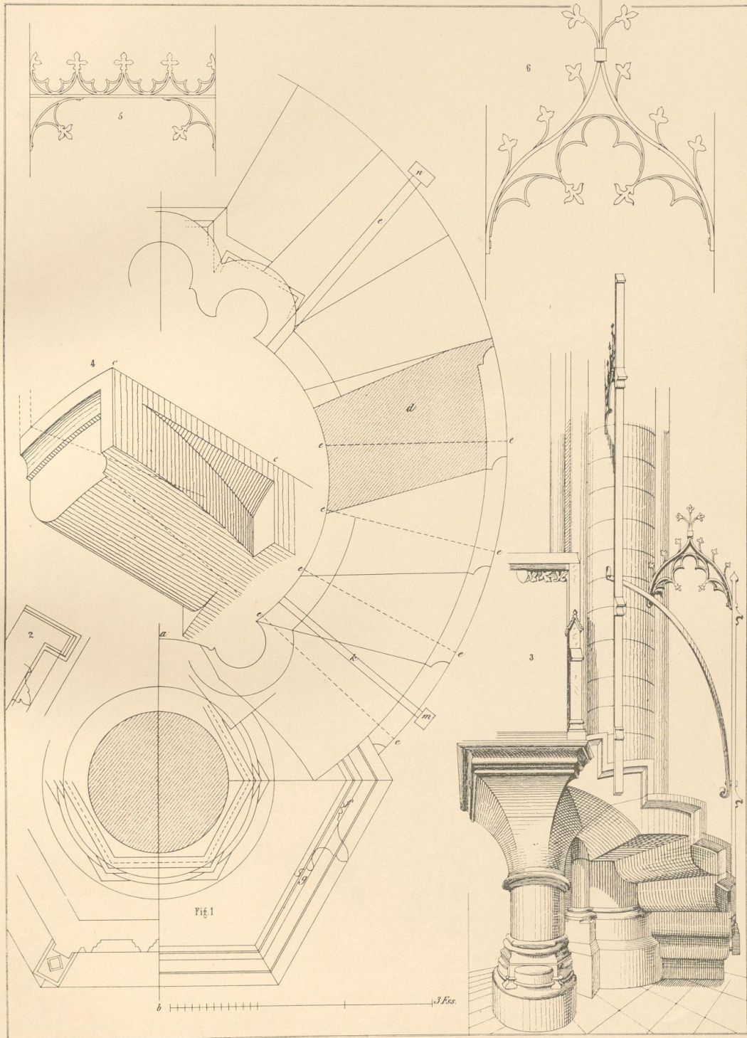
Kanzel aus der Kathedrale zu Besancon (vgl. Taf. 89).
