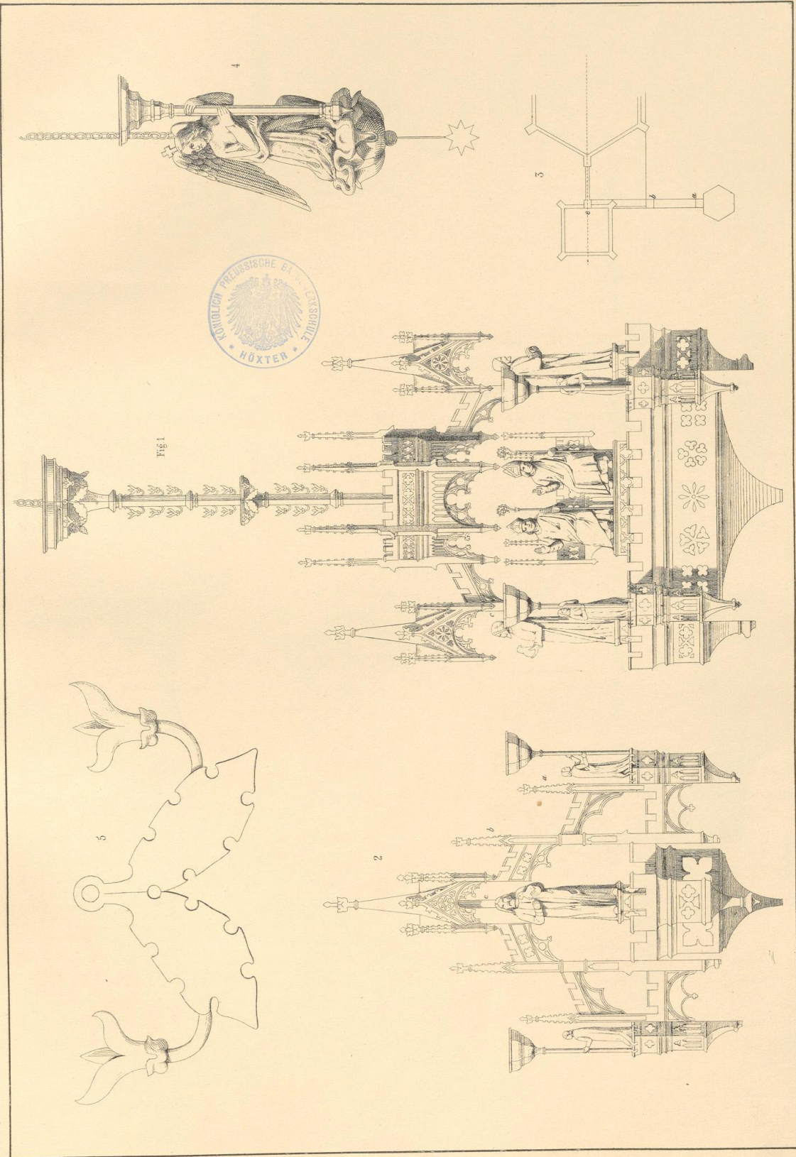
Hängeleuchter aus Kupfer aus dem Dome in Eibstedt.
