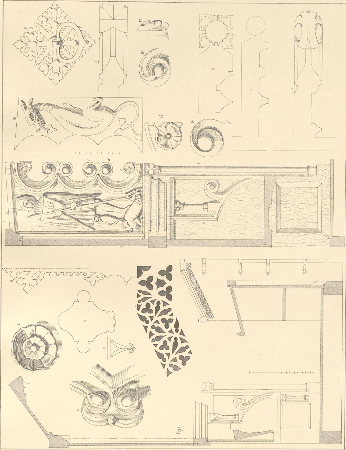
Eingebauten vom Chorgesäß aus Sülzkanten (siehe Tafel 119).
