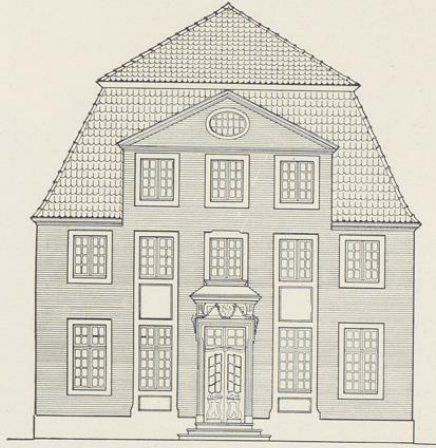
Abb. 1131. Aufriß der Front des Hauses Loerstraße 1 Dachhaus von 1779; Maßstab 1 : 200
