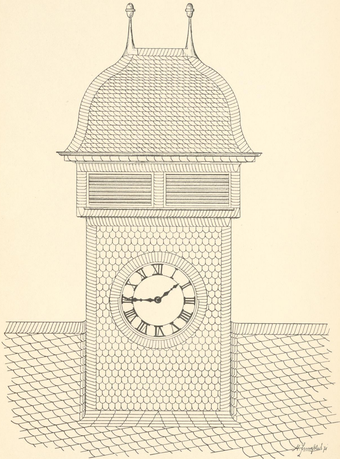
Dachreiter mit Schuppenschablonen, Rundplättchen und Schrägorsteinen.
