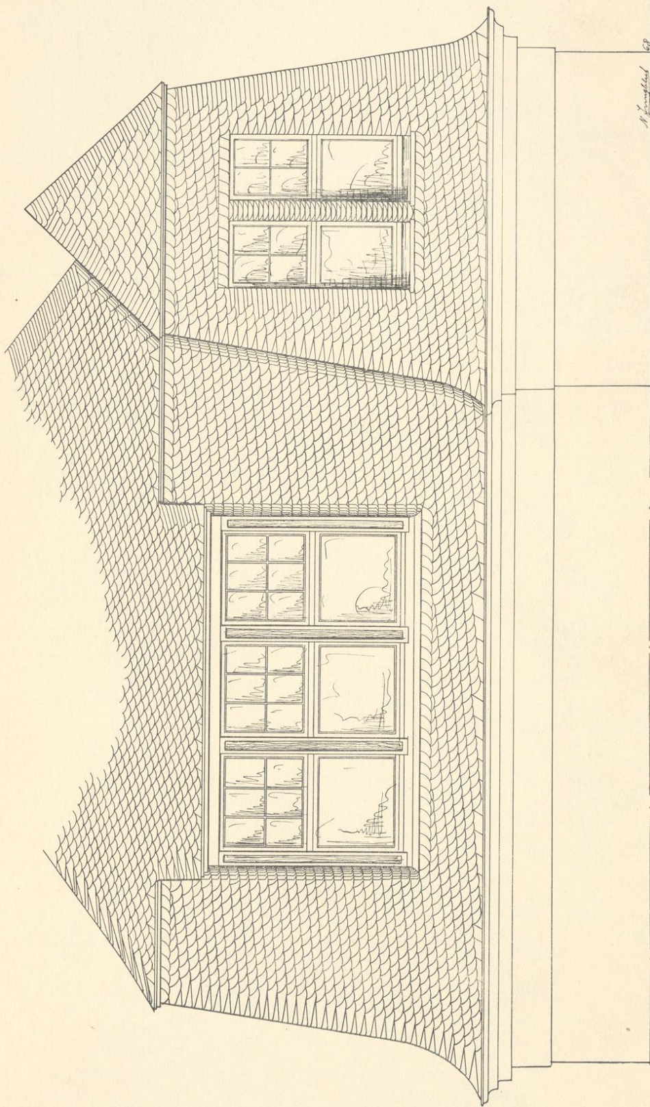
Mansarde mit Vorbau, deutschem Recht- und Linkort. Kehlen eingehend gedeckt.
