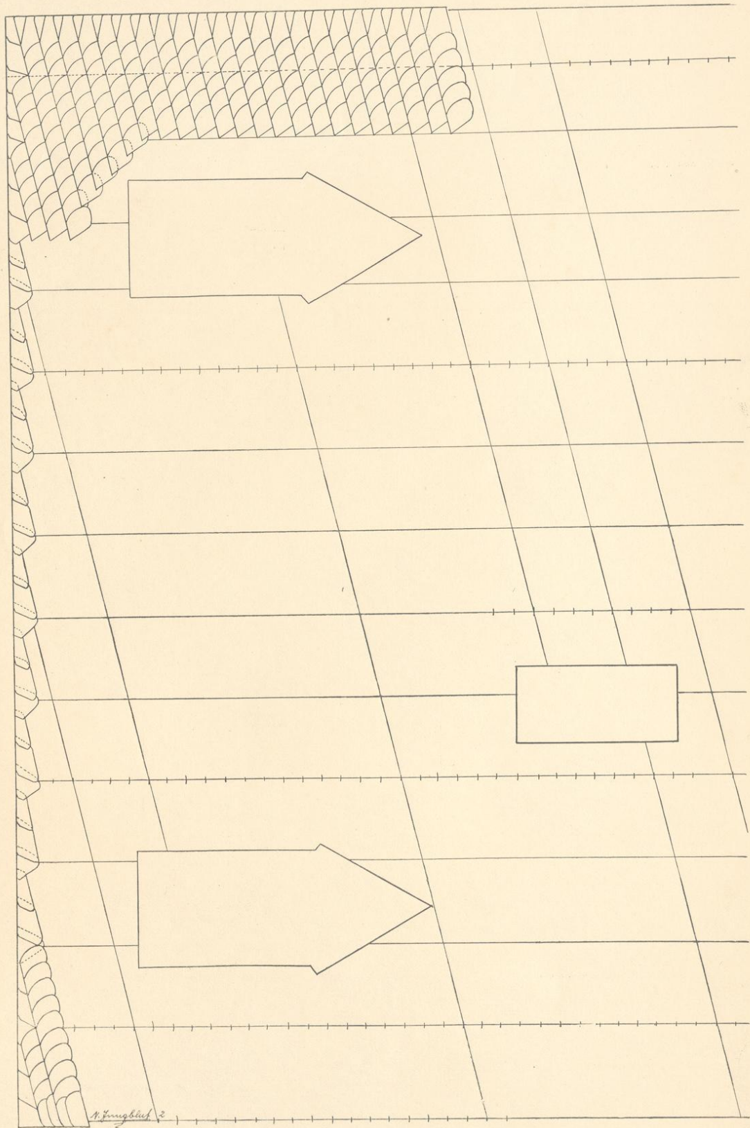
Deutsche Deckung mit Schuppenschablonen.
