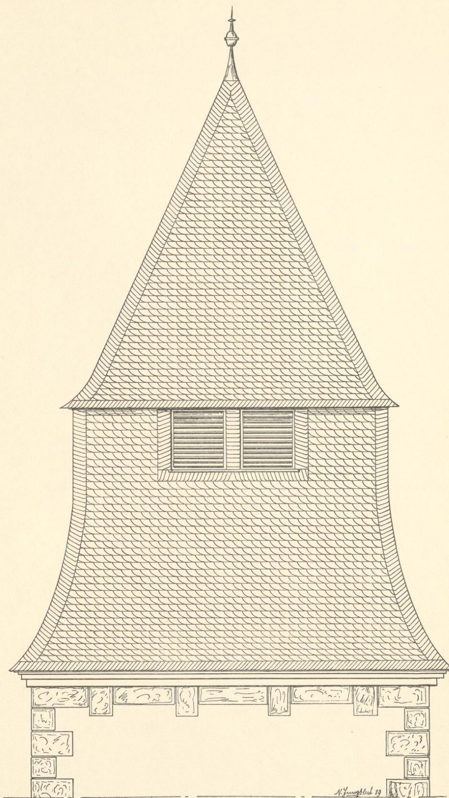
Turm mit Vertikalschuppen ohne Steigung und Strackort. Vergl. mit Blatt 90 und 91.
