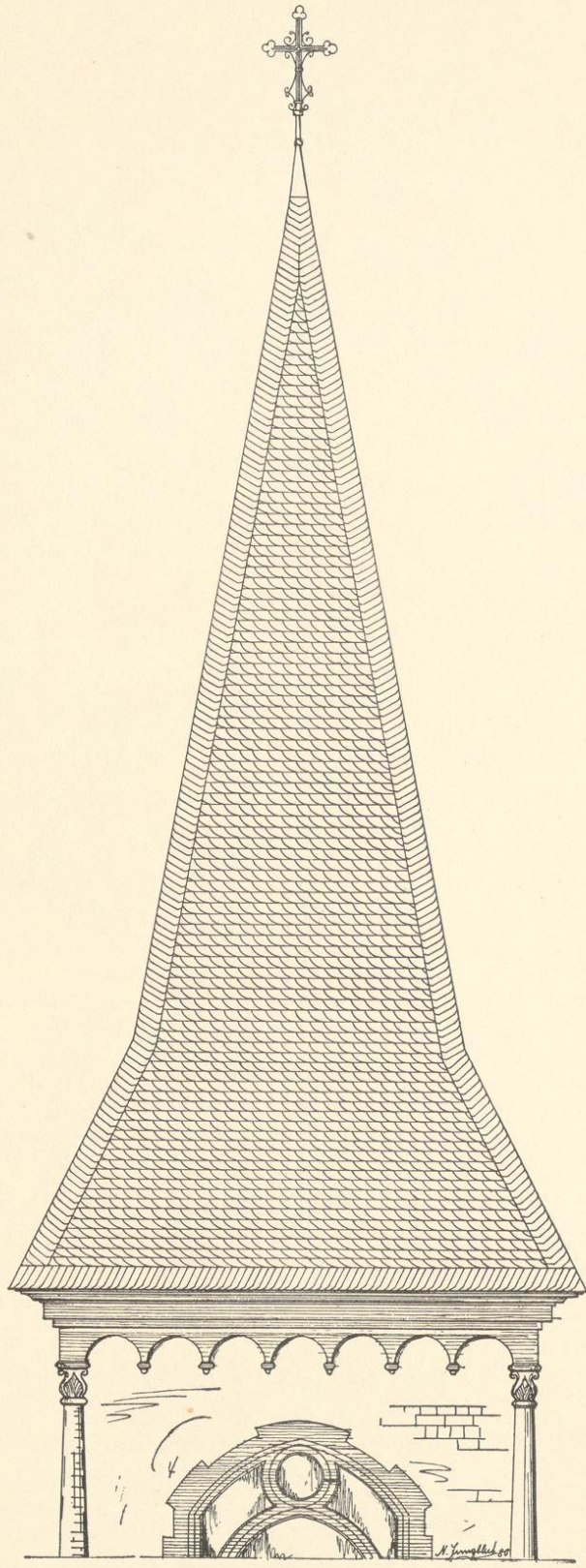
Kirchturm mit Vertikalschuppen ohne Steigung. Strackort mit Schrägortsteinen.
