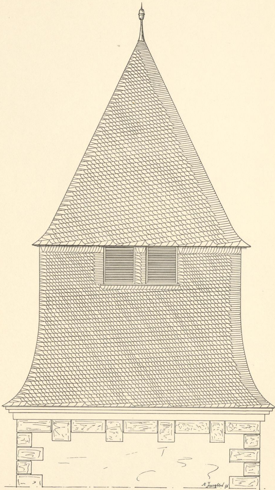
Turm wie Blatt 89 und 90 jedoch in altdeutscher Deckung.
