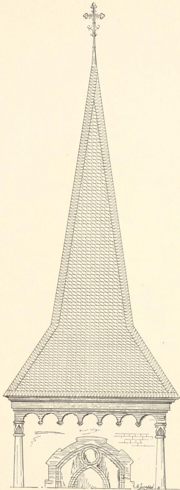
Kirchturm wie Blatt 80 mit Wechselort.
