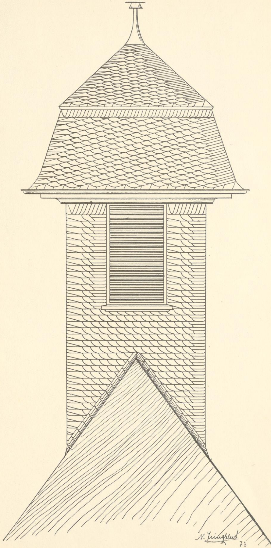
Dachreiter. Giebelansicht zu Blatt 72.
