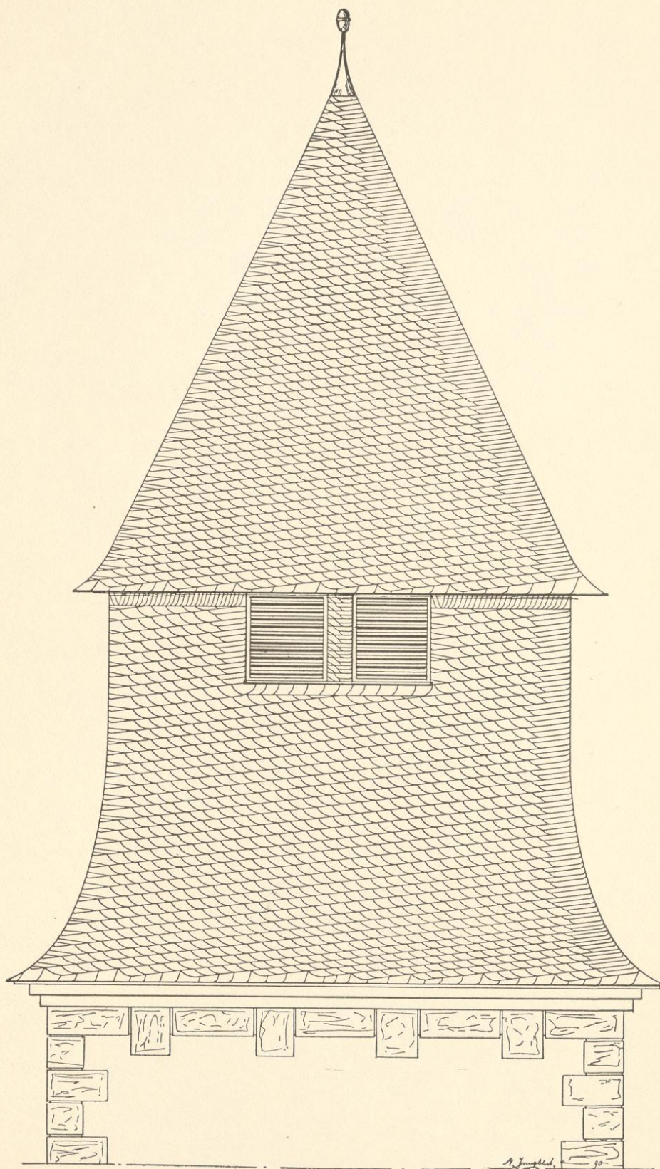
Turm wie Blatt 89 jedoch mit Steigung und deutschem Recht- und Linkort.
