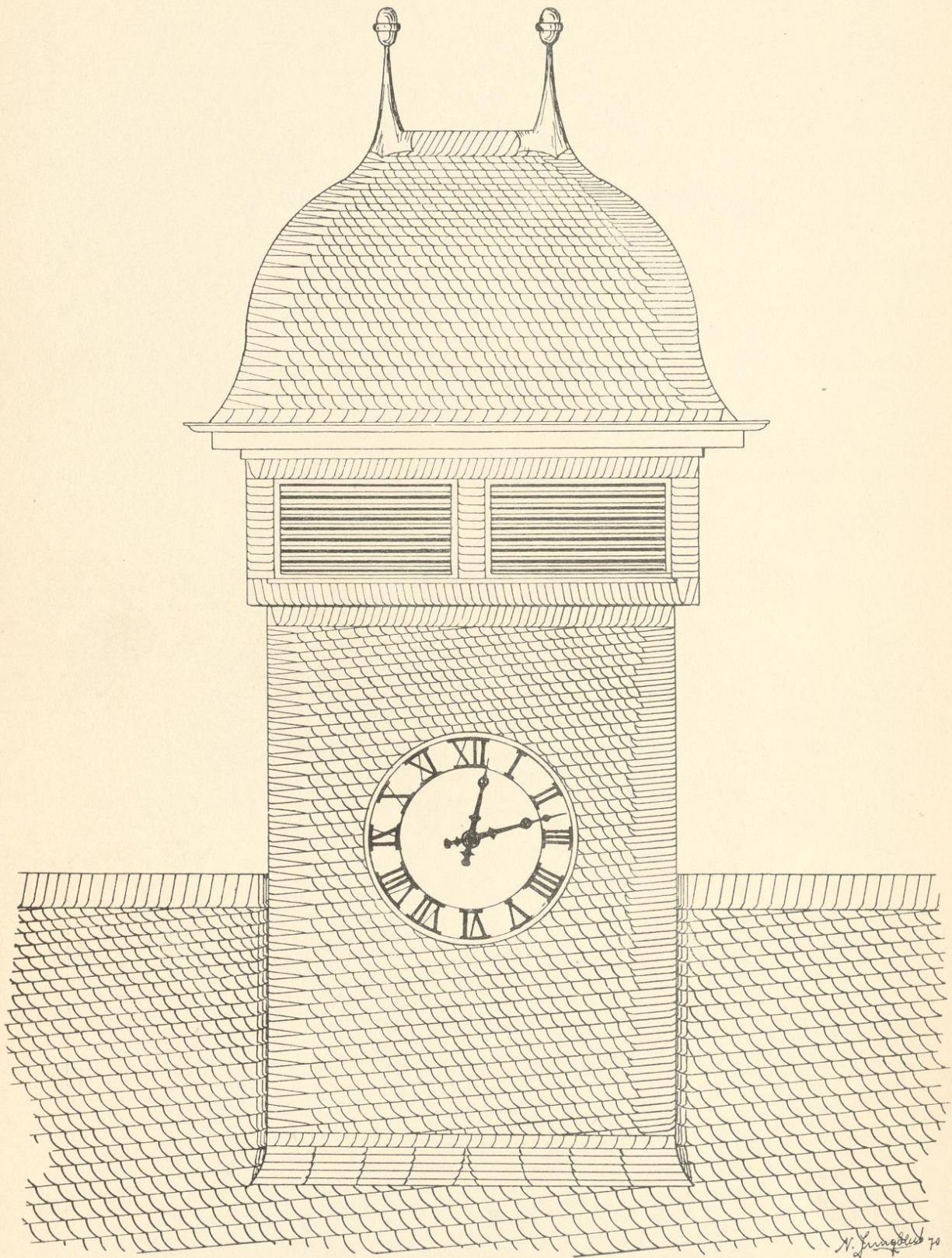
Dachreiter in altdeutscher Deckung Wandfläche mit Steigung.
