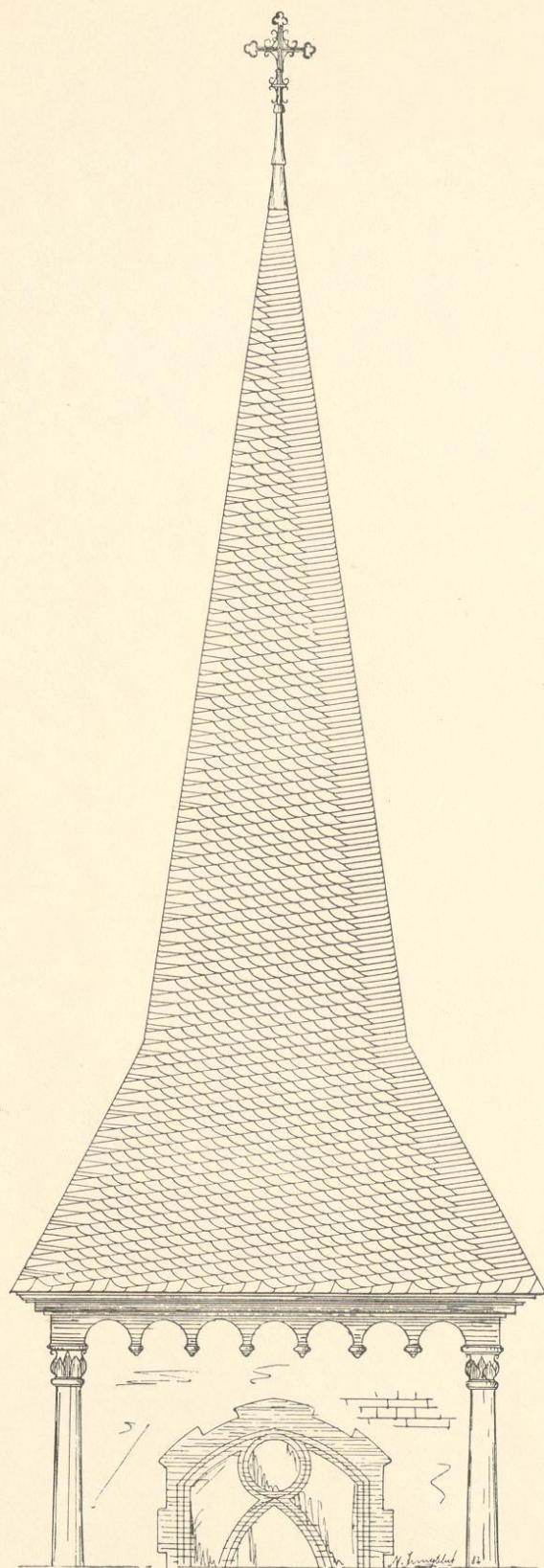
Kirchturm wie Blatt 81 jedoch mit Steigung und deutschem Recht- und Linkort. Rechtort gleichmäßig gehalten,
