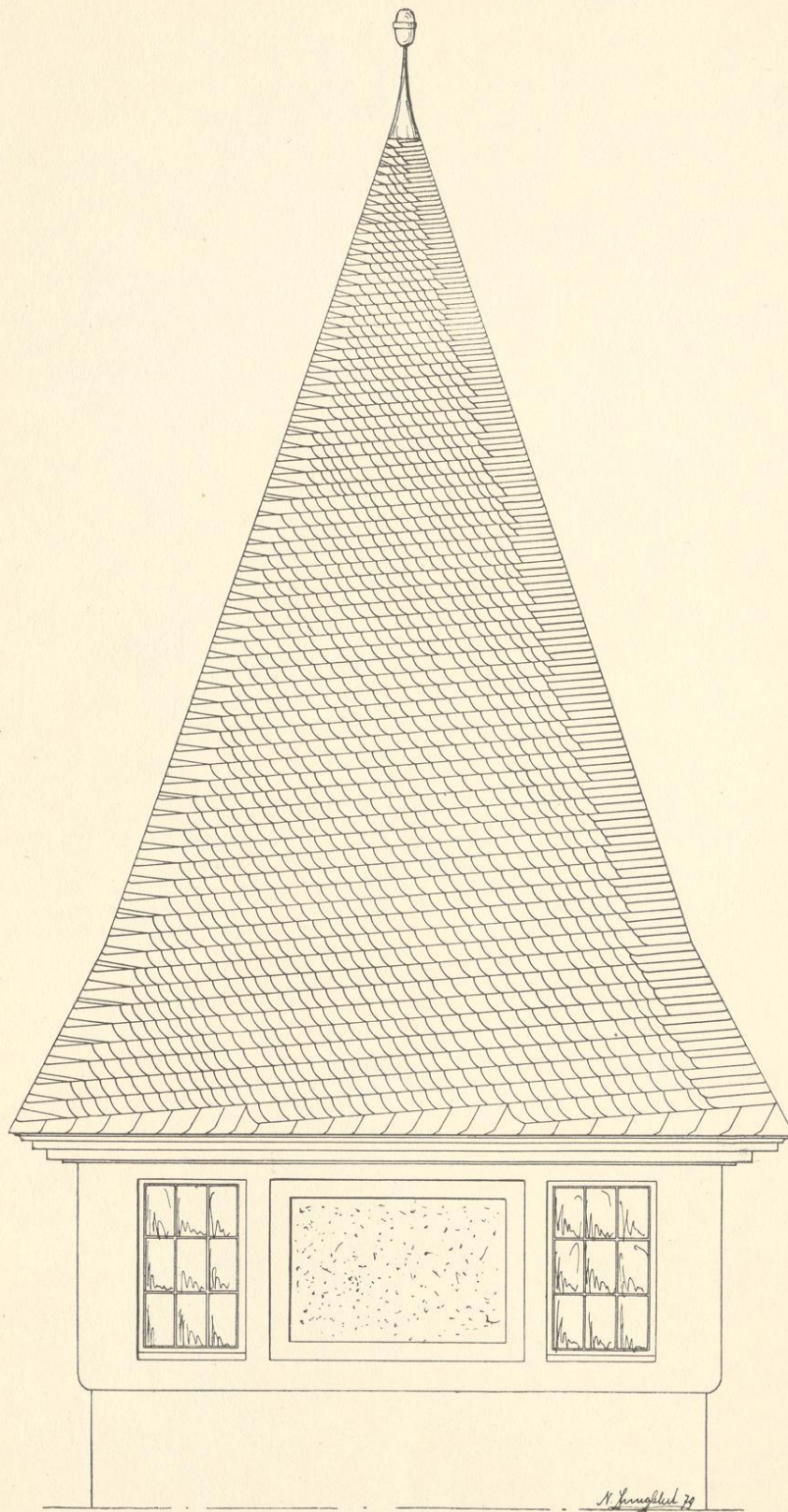
Turm in altdeutscher Deckung.
