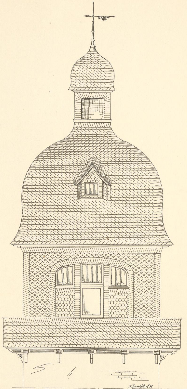
Kuppelturm mit Veranda. Vertikalschuppen, Fischschuppen, Rundplättchen, Recht- und Linkstichort.
