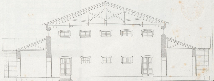
Durchschnitt nach A. B.
