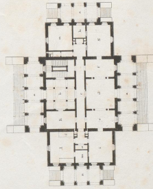
Grundriss des ersten Stockes
