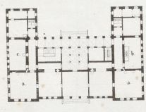
Grundriss des A: Der Saal B: Die Bibliothek, die Schreibstube und die Kanzlei C: Die Kassen und die Verwaltung
