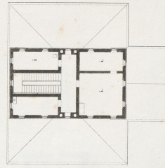
B. Grundriss der oberen Stocke.
