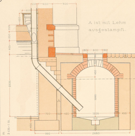
Schnitt AB.
