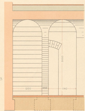
Schnitt JK.
