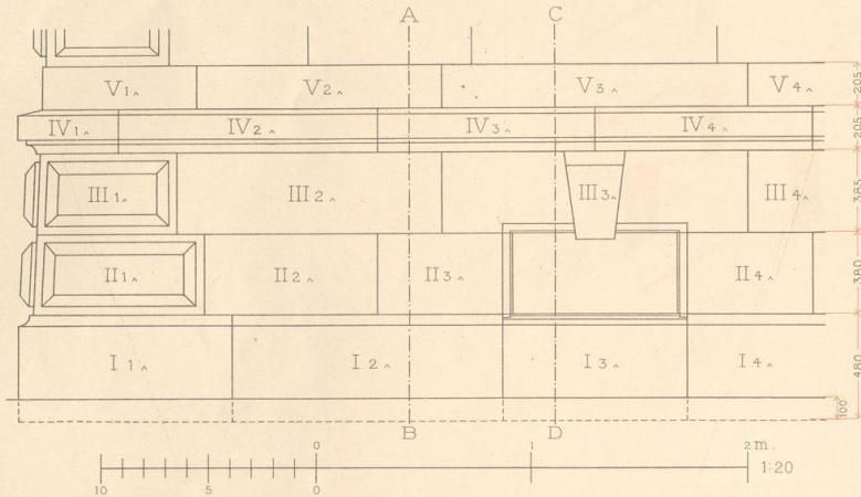
Ansicht der westlichen Ecke des Wohnhaussockels.
