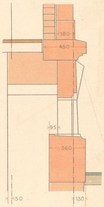
Schnitt C D.
