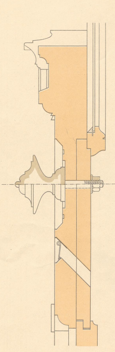
Schnitt ab.
