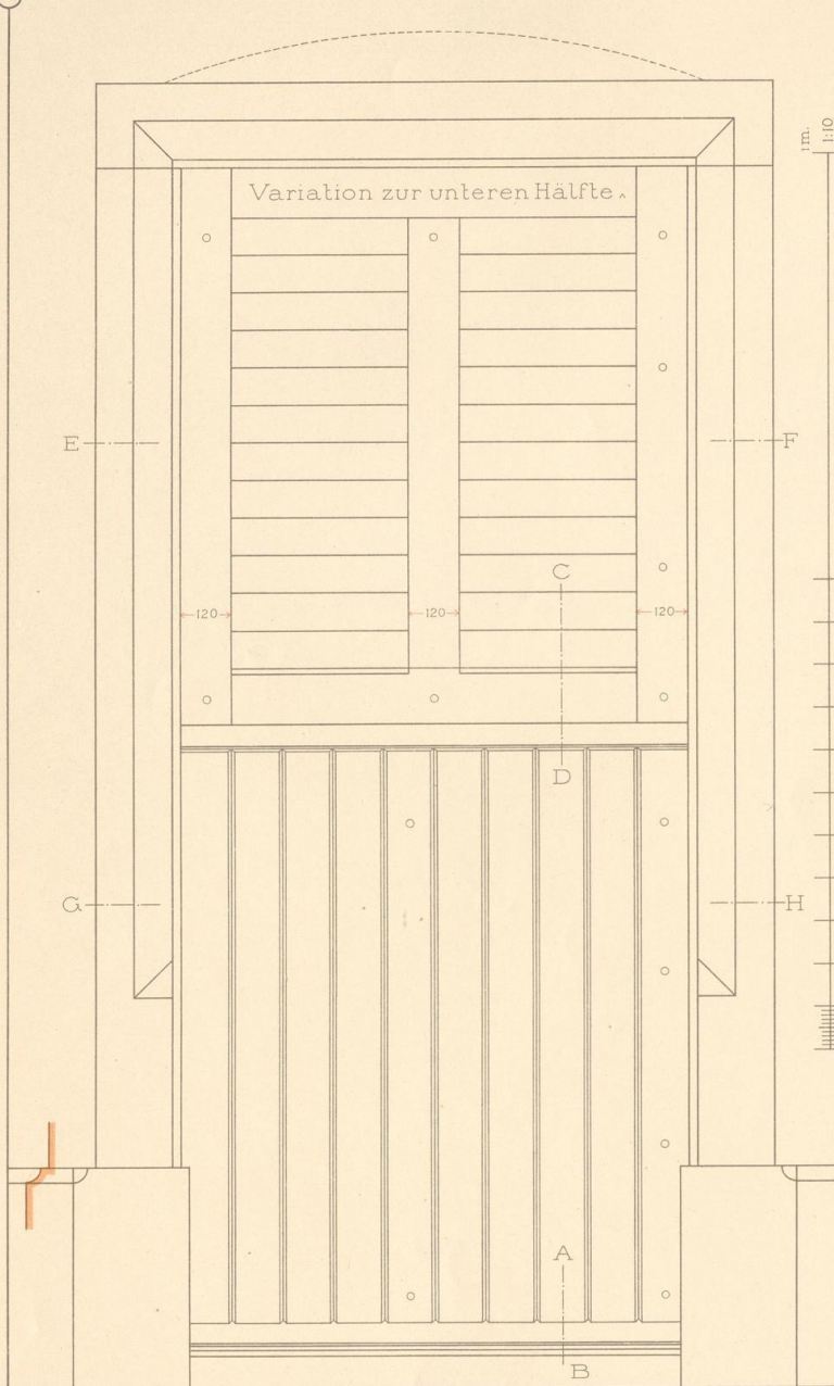
Aussere Ansicht.
