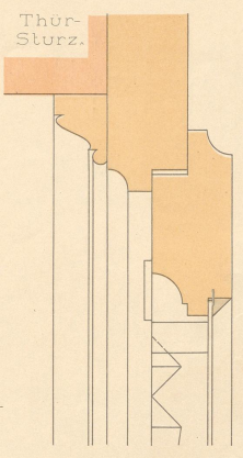
oberer Schnitt.
