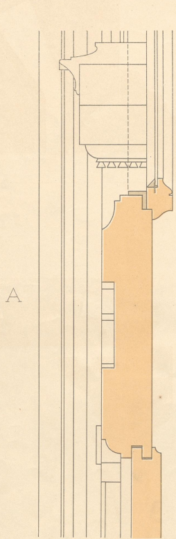
Schnitt durch den untern Teil der Thüre.
