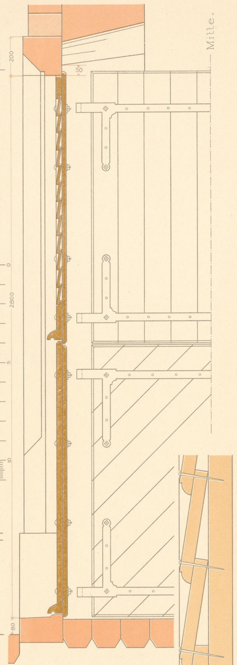
Schnitt u. innere Ansicht.
