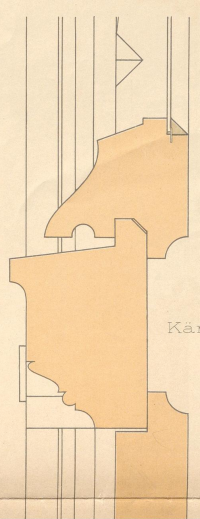
oberer Schnitt.
