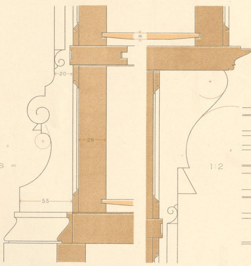
Schnitt ab.
