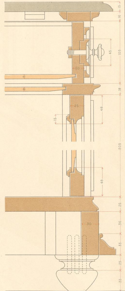
Schnitt e f.
