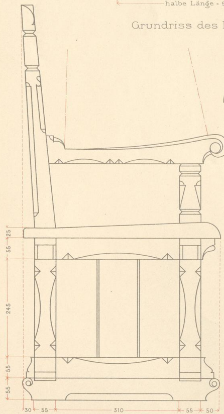
Seitenansicht.
