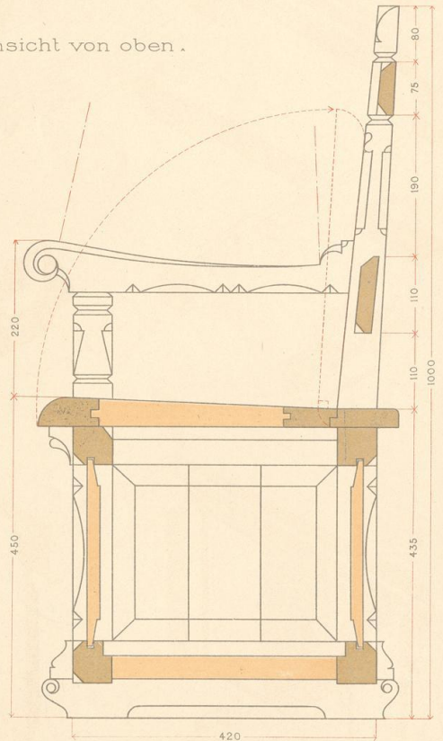
Querschnitt.
