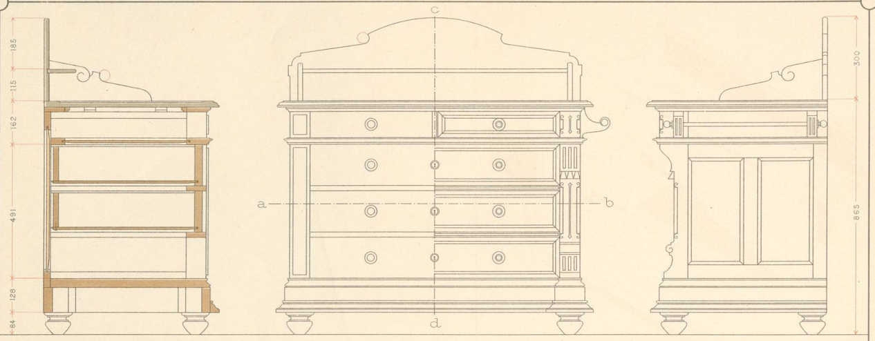
Schnitt c d.
