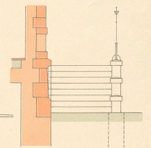
Schnitt C D.
