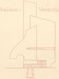
Schnitt C D.
