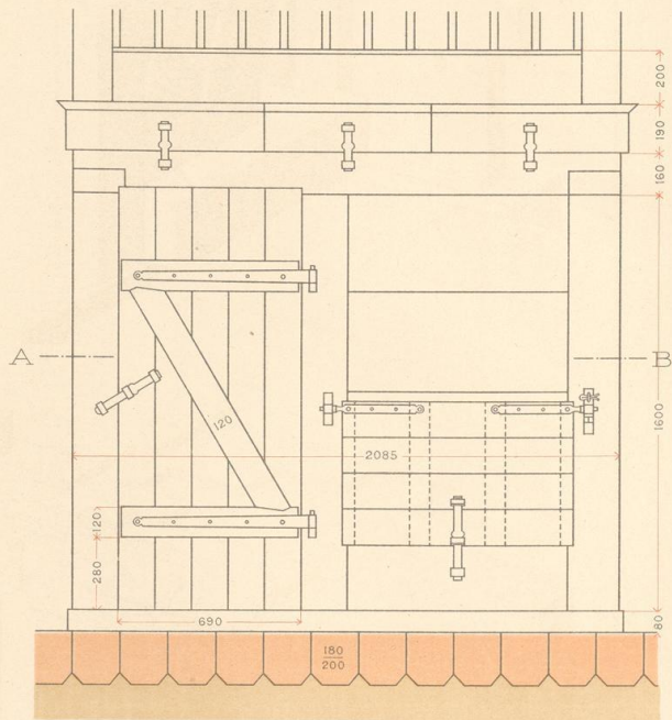
Ansicht.
