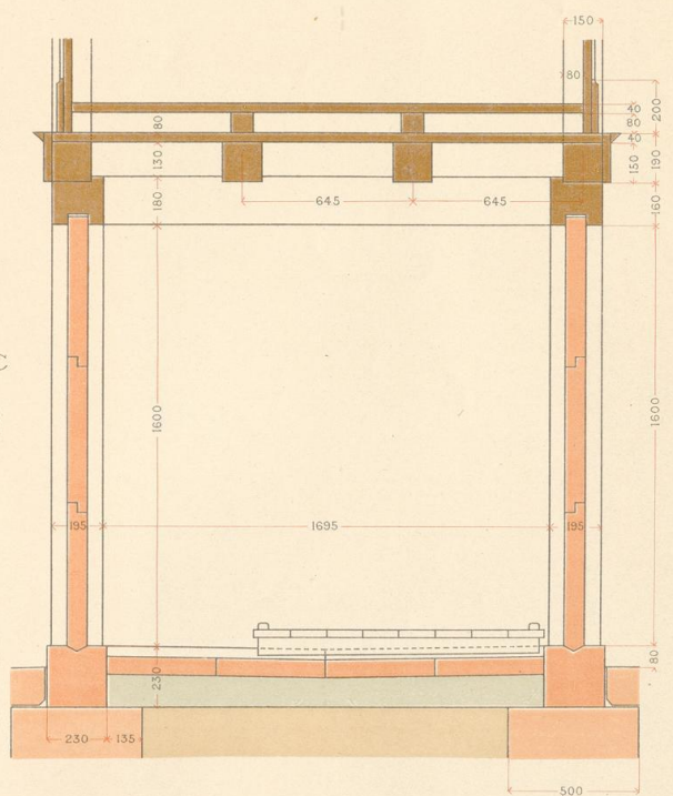
Schnitt BC.
