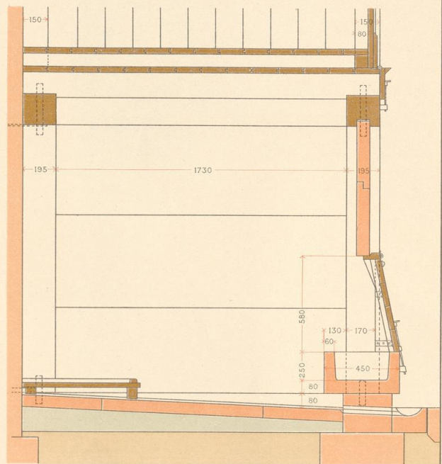
Schnitt CD.
