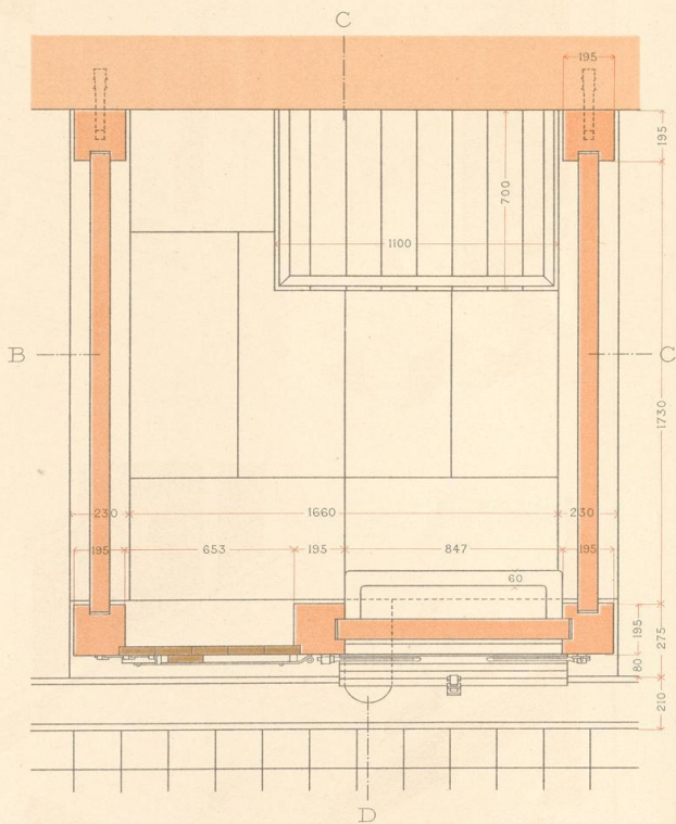
Schnitt AB.
