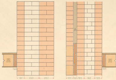
Die Zwischenräume A sind ausgemauert.
