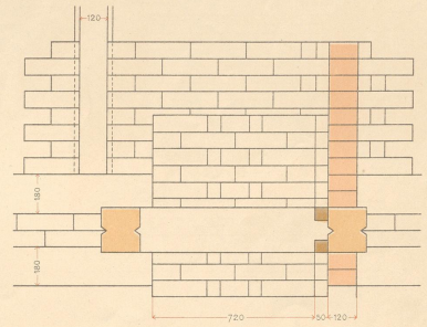
Die Zwischenräume A sind ausgemauert.
