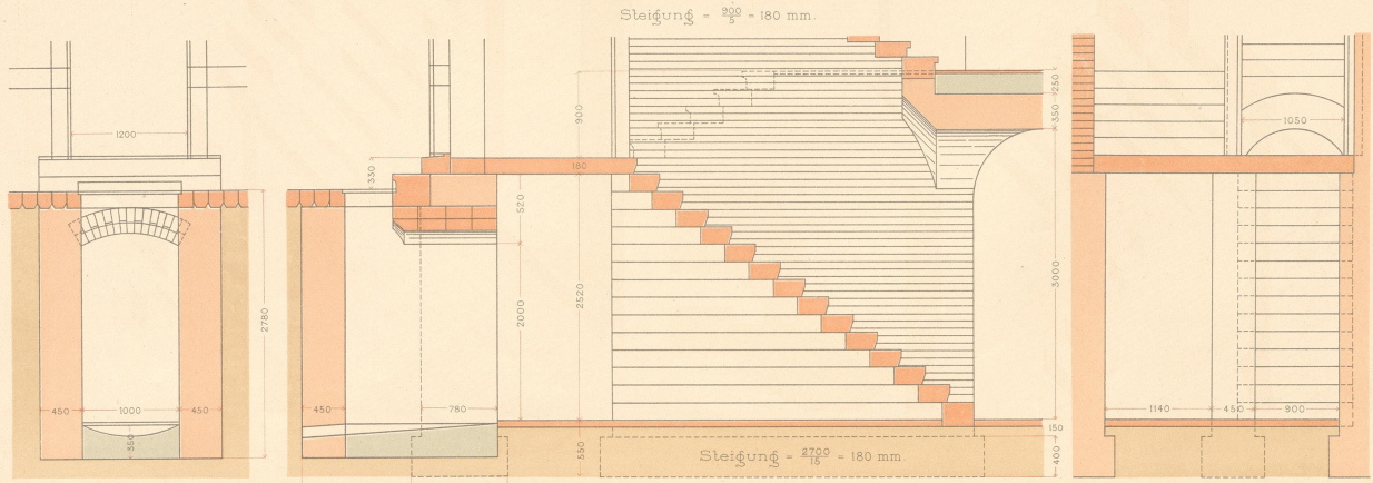
Schnitt CD.
