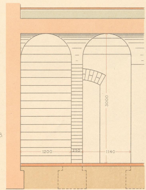
Schnitt JK.
