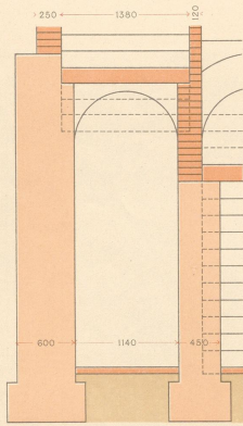
Schnitt GH.
