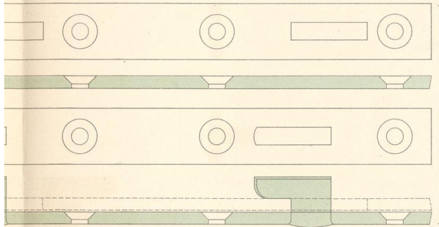
Beschläge nat Gr.
