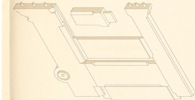
Dübelung der Frese.
