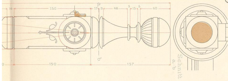
Beschläge nat Gr.
