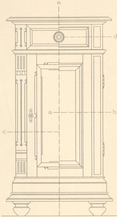
Vorderansicht.
