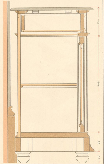
Schnitt ef.
