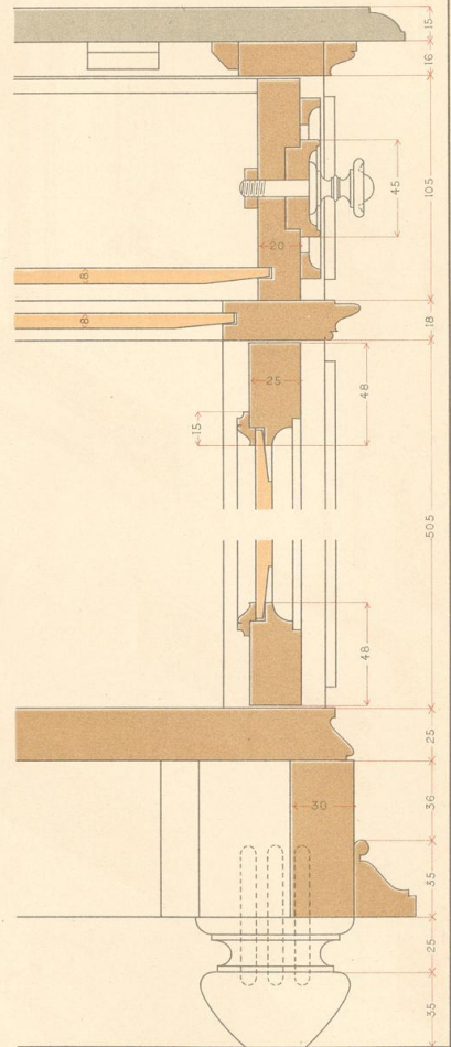
Schnitt ef.
