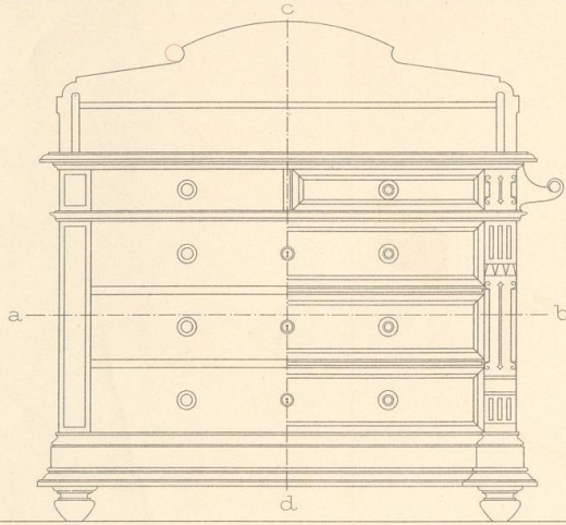
Vorderansicht.
