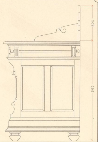
Seitenansicht. Variation.
