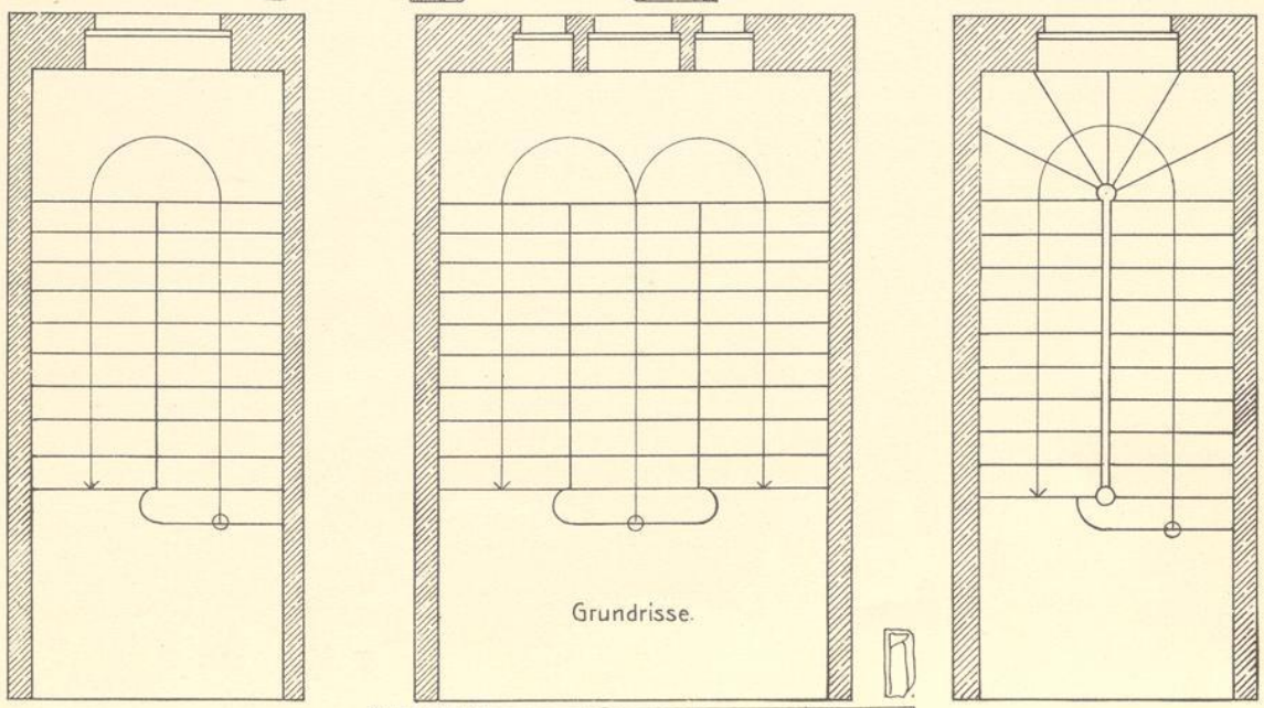
Treppen.
