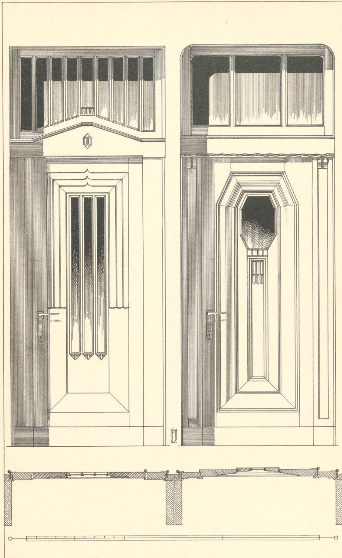
Einflügelige Haustüren.
