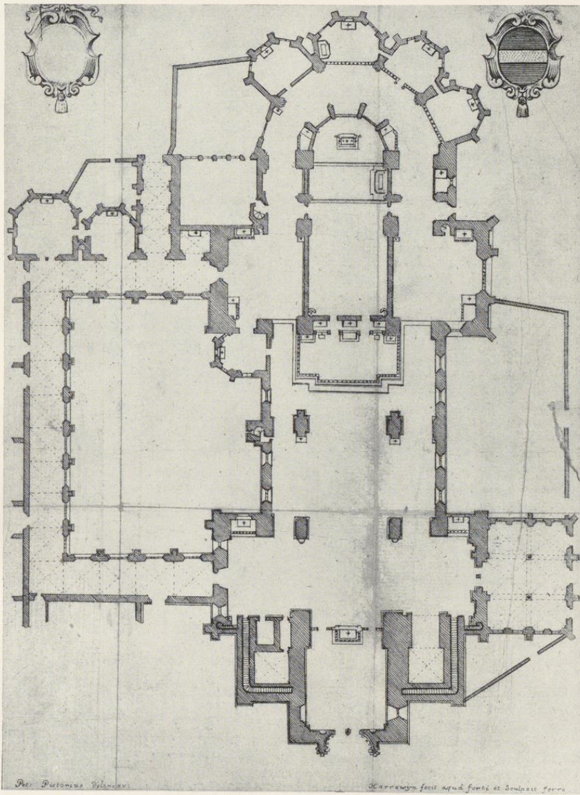
Abb. 1371. Grundriß des Domes um 1710. Radierung von J. Harrewyn nach Peter Pictorius d. J., aus Histoire ecclésiastique d'Allemagne . Brüssel 1724. Vgl. S. 11, 3.
