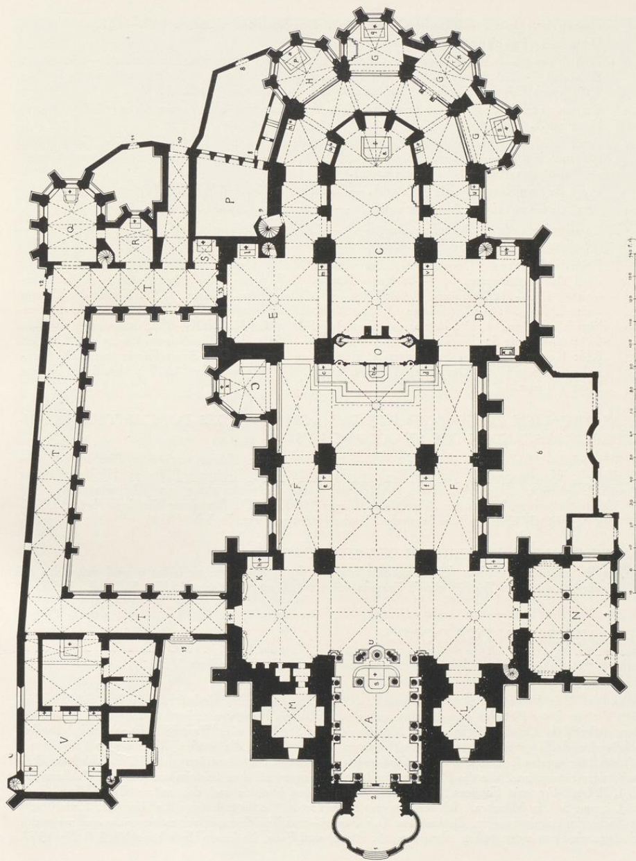
Abb. 1373. Grundriß des Domes, vermutlich von van der Giese 1761, kopiert 1831. Norden oben. Staatsarchiv Nr. 879. Vgl. S. 11 Nr. 6; die Erläuterung der Buchstaben und Zahlen auf S. 13
