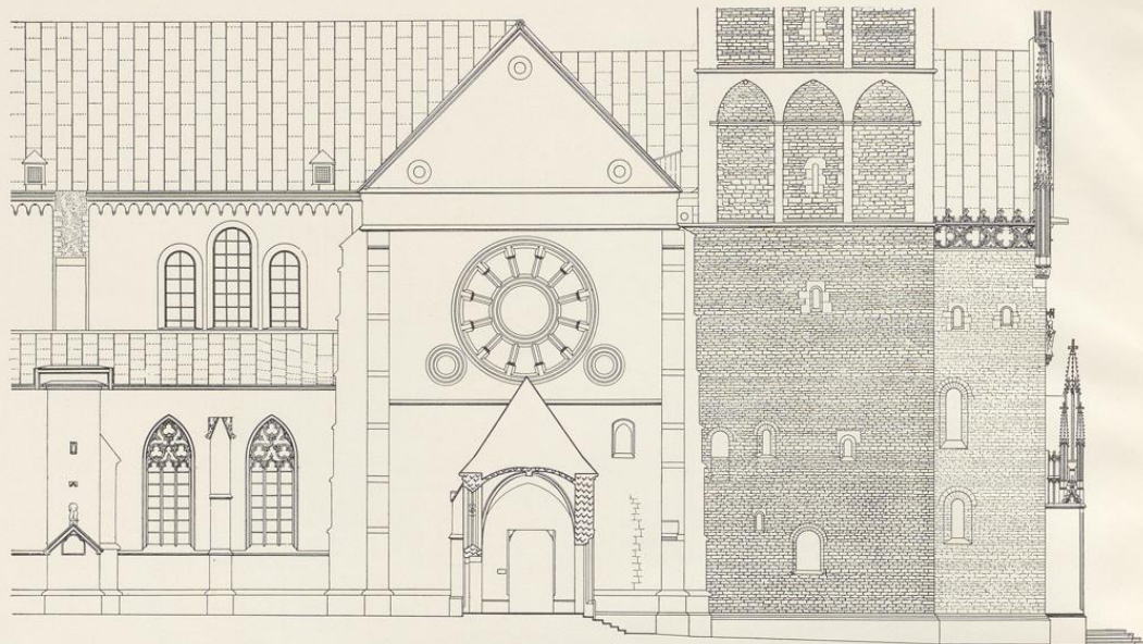
Abb. 1705. Aufriß der westlichen Hälfte der Nordseite; Maßstab 1 : 300
