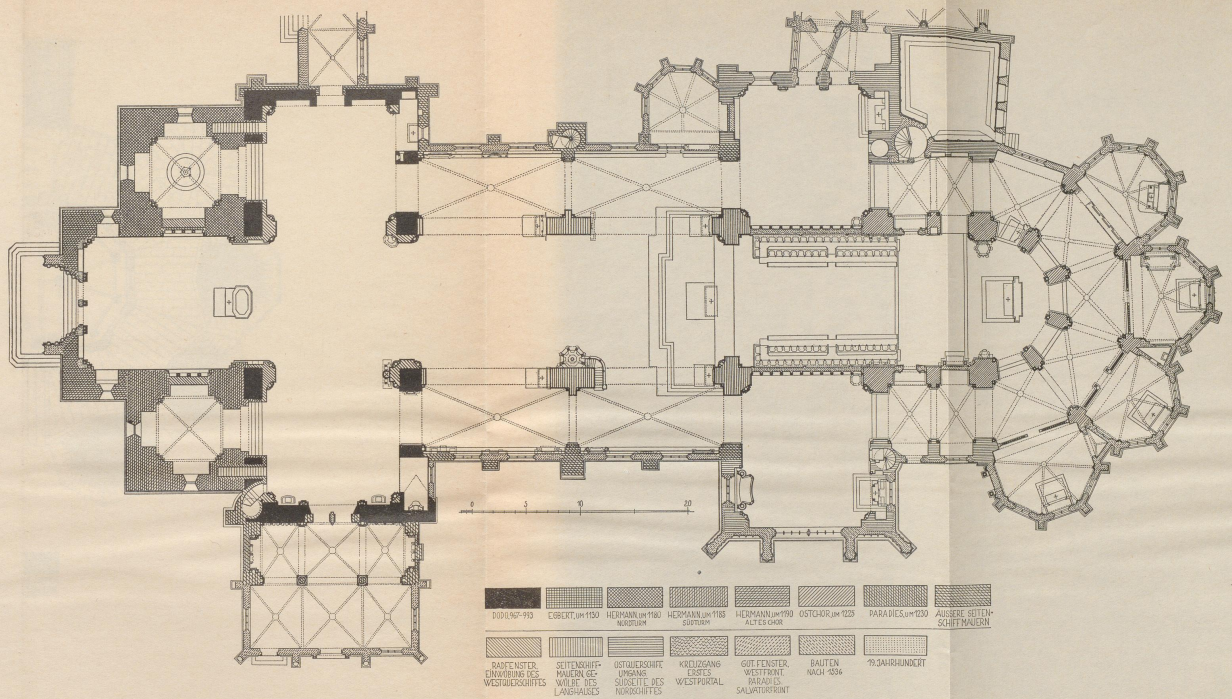
Abb. 1694. Grundriß des Erdgeschosses; Maßstab 1:300
