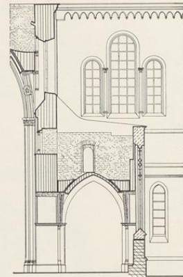
Abb. 1712. Schnitt des nördlichen Seitenschiffes, Westjoch nach Westen
