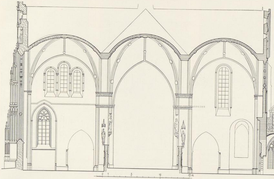
Abb. 1714. Schnitt des Ostquerschiffes nach Westen
