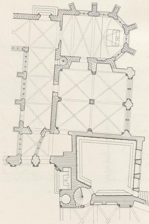
Abb. 1717 (unten) Grundriß der Marien- kapelle, der neuen Sakristei und des Kapitelsaales
