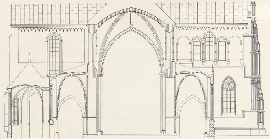
Abb. 1713. Schnitt des Hochschiffes und der Seitenschiffe, östliche Joche, nach Osten Maßstab 1 : 300
