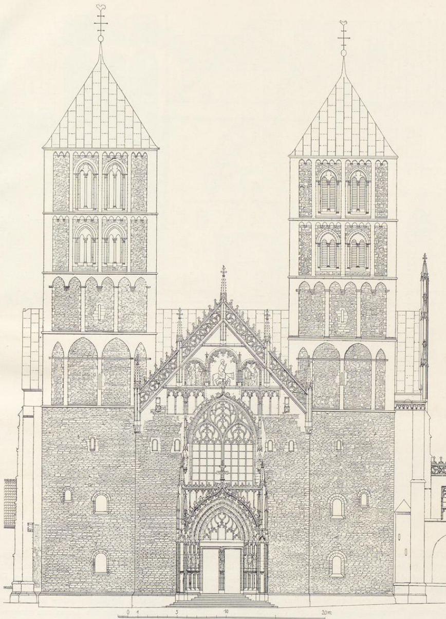
Abb. 1704. Der Aufriß der Westfront; Maßstab 1 : 300
