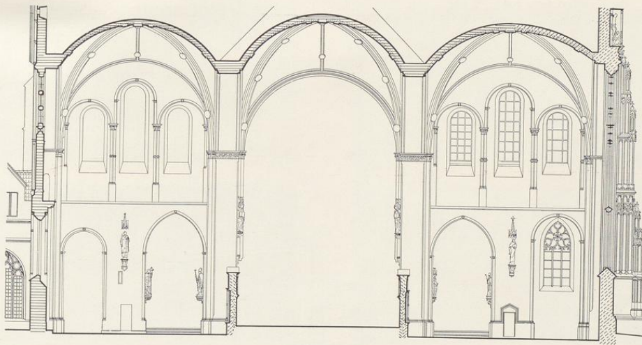
Abb. 1715. Schnitt des Ostquerschiffes nach Osten
