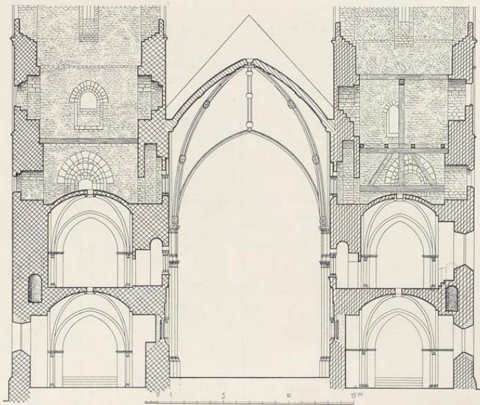
Abb. 1708. Schnitt durch das Westwerk nach Osten; links der Nordturm
