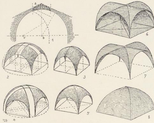
Abb. 1699. Veranschaulichung der Domikalgewölbe mit vertieften Diagonal- und Kreuzrippen
