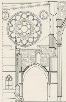
Abb. 1711. Schnitt des südlichen Seitenschiffes, Westjoch nach Westen
