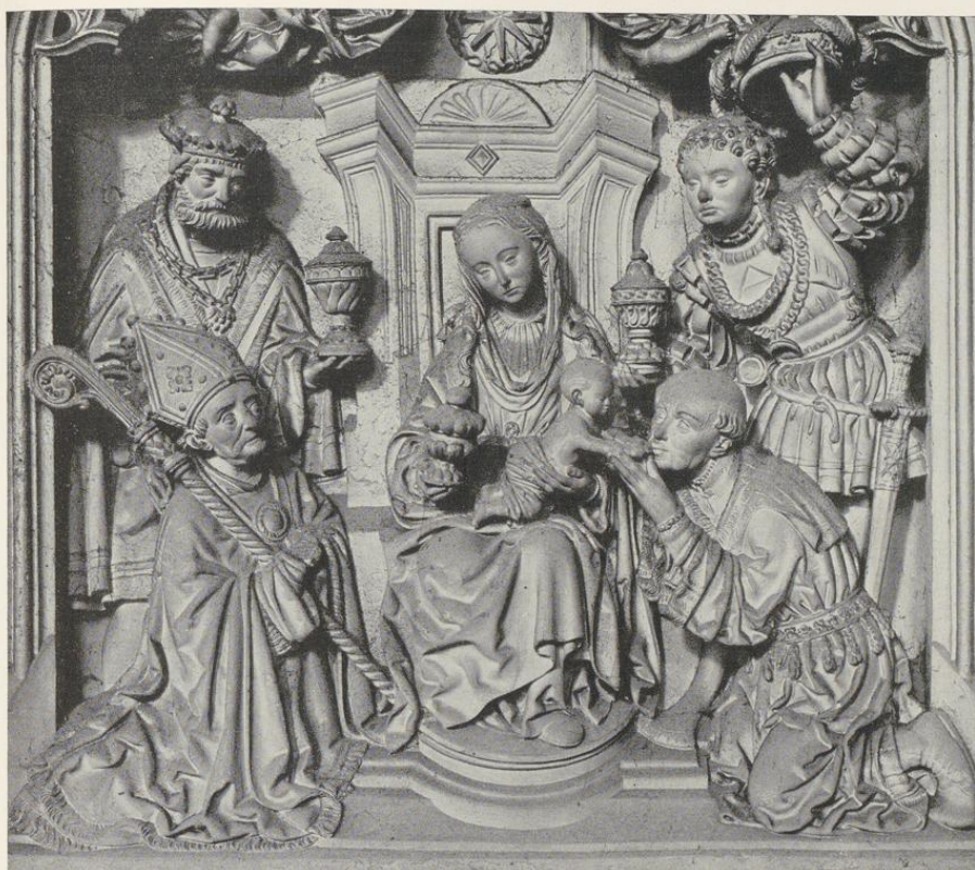
Abb. 1516. Einzelaufnahme des Epitaphs des Weihbischöfs Johann Bischopink von Johann Brabender. Vgl. S. 258
