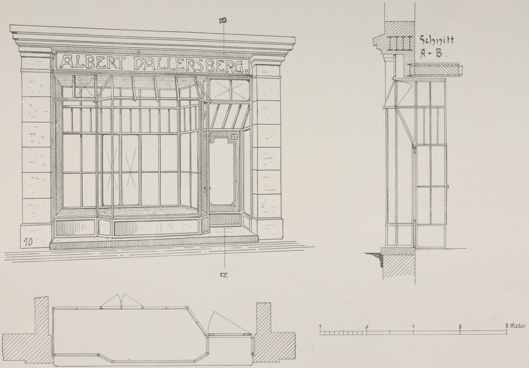
Schaufensteranlage mit in der Mitte vorgebautem Schaufenster und seitlichem Eingang
