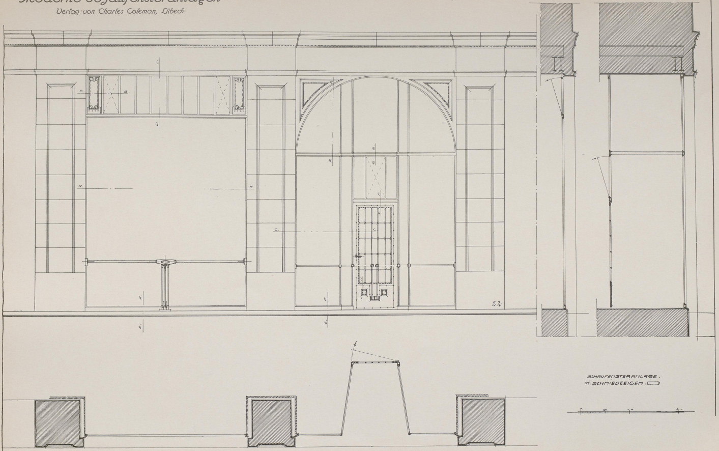
Schaufensteranlage in Schmiedeeisen mit einem einfachen Fenster und einem Doppelfenster mit Türeingang Konstruiert von S. Wälten, Hamburg
