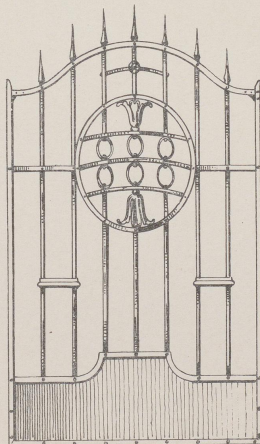
Einhäng- bezw. versenkbare Gitter für Schaufenster-Anlagen Konstruiert von O. Starke, München
