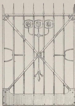
Maßstab 1 : 20
