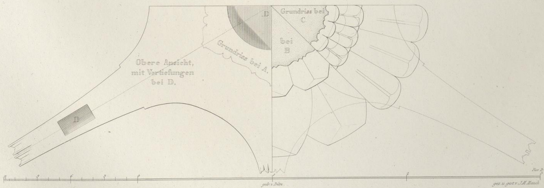
DIE BEKRÖNUNG, DES CHORAGISCHEN MONUMENTS DES LYSIKRATES IN ATHEN.
